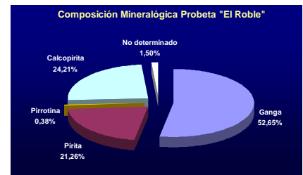
Figura 2. Composición Mineralógica (% de Áreas).
