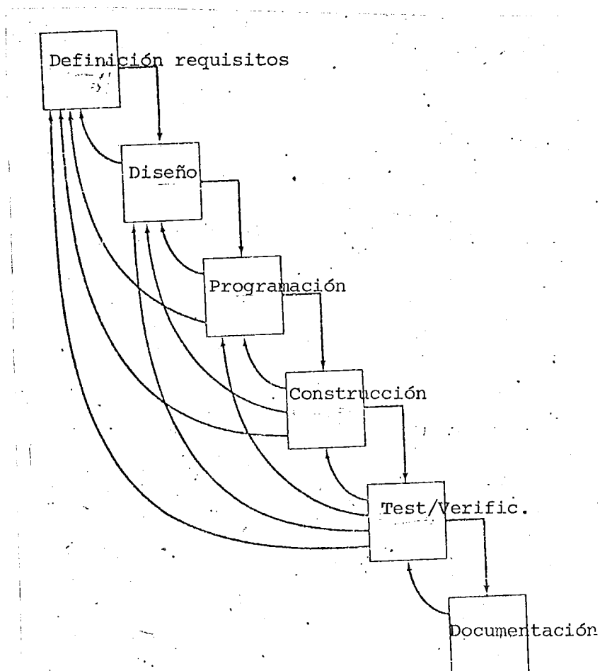
FIG. 13 INTERRELACION DE LAS ETAPAS DEL PROCESO DE DESARROLLO PARA GRANDES SISTEMAS, SEGUN (FOX, 1982)
