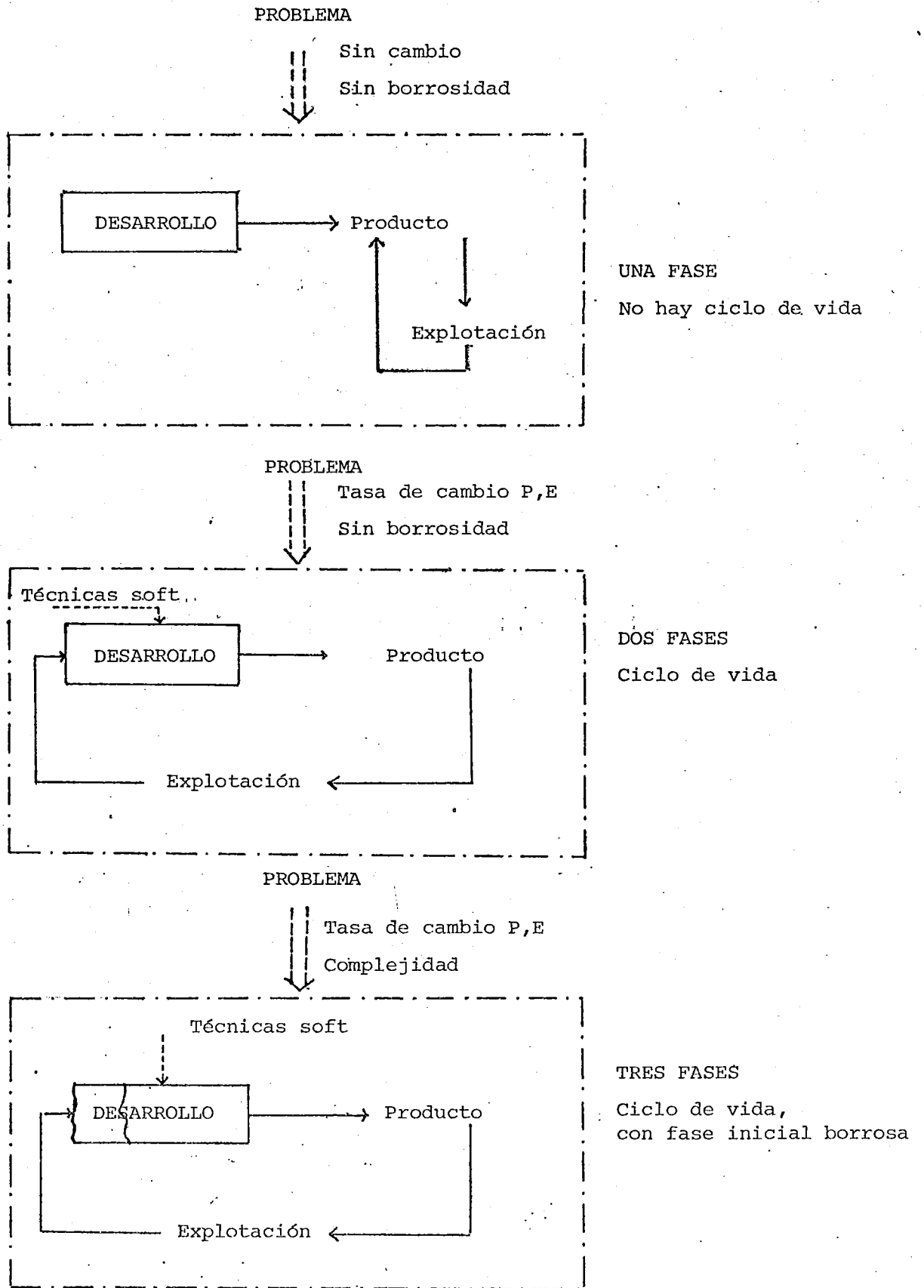
Fig. 8. RESUMEN DE ENFOQUES DEL PROCESO DE DESARROLLO (INFLUENCIAS DE LA NATURALEZA DEL PROBLEMA)
