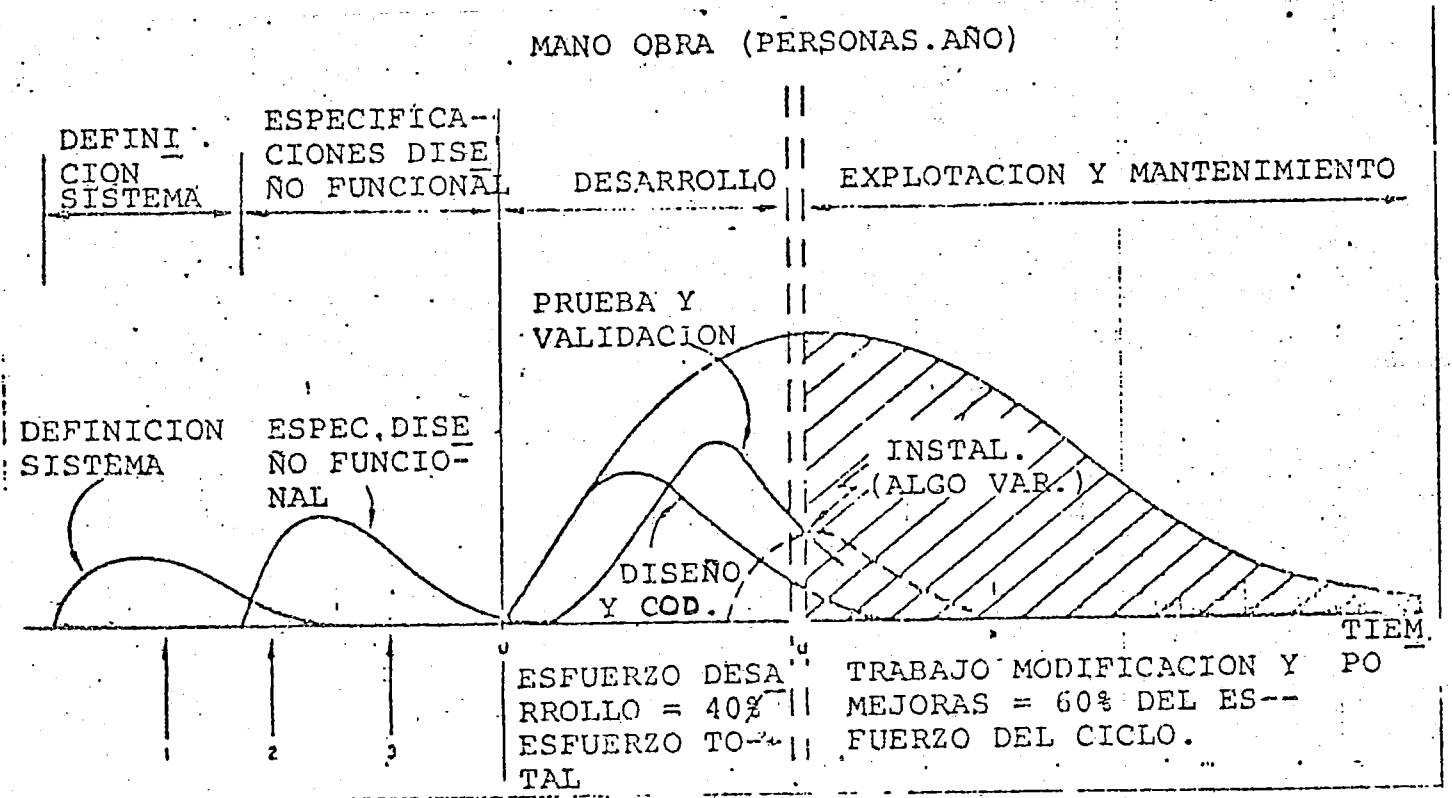
FIG. 9. CURVA DE RAYLEIGH.
