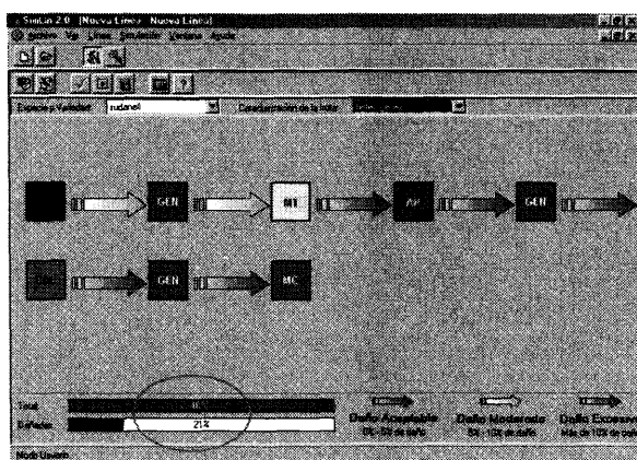
Figura 1. Ejemplo de simulación de daños en la línea 3 cuando manipula melocotón de la variedad Sudanell. La caracterización de la fruta cuyos resultados se muestran (21% de frutos dañados) es la denominada heterogénea y refiere a frutos con una firmeza Magness-Taylor media de 20N + 6N. Las flechas amarillas indican porcentajes de fruto dañado superiores al 5% e inferiores al 10%.
