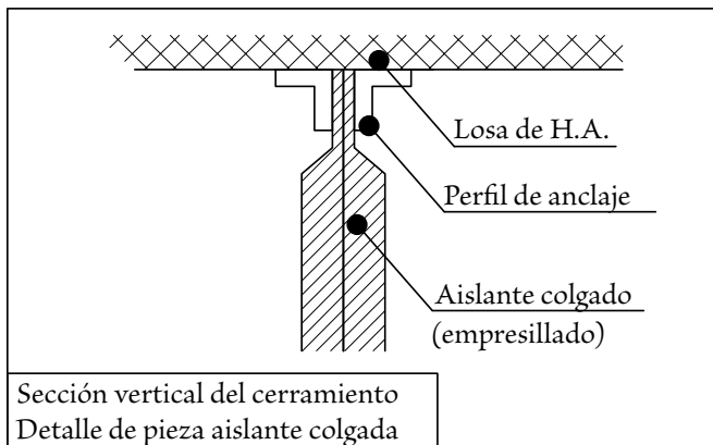
(14) Detalle constructivo 3
