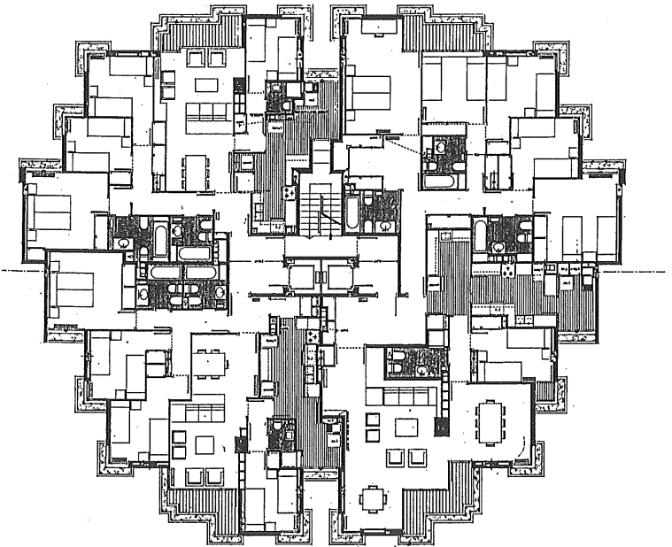
J. A. Coderch: Planta del edificio Girasol, Madrid, y planta de una unidad en el conjunto de cocheras, Barcelona.
