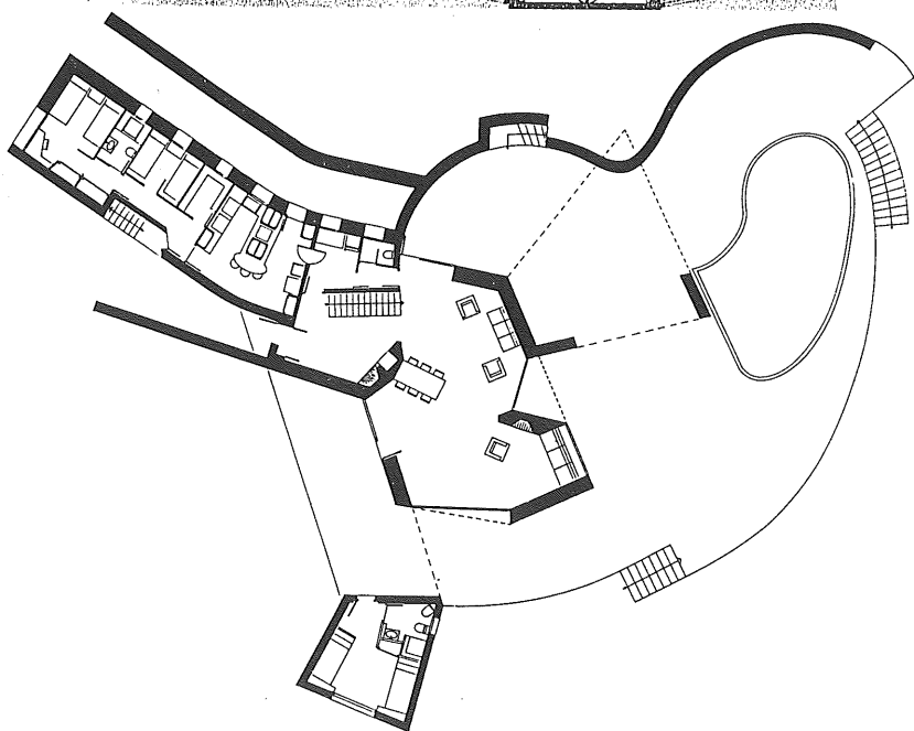
J. A. Coderch: Planta del edificio de viviendas la La Barceloneta y planta de la Casa Ugalde en Caldetas.
