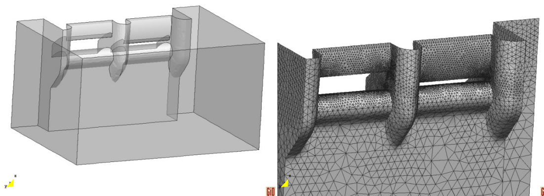
Figura 3 Geometría de uno de los casos. Izquierda: vista general; derecha: detalle de la malla de elementos finitos.
