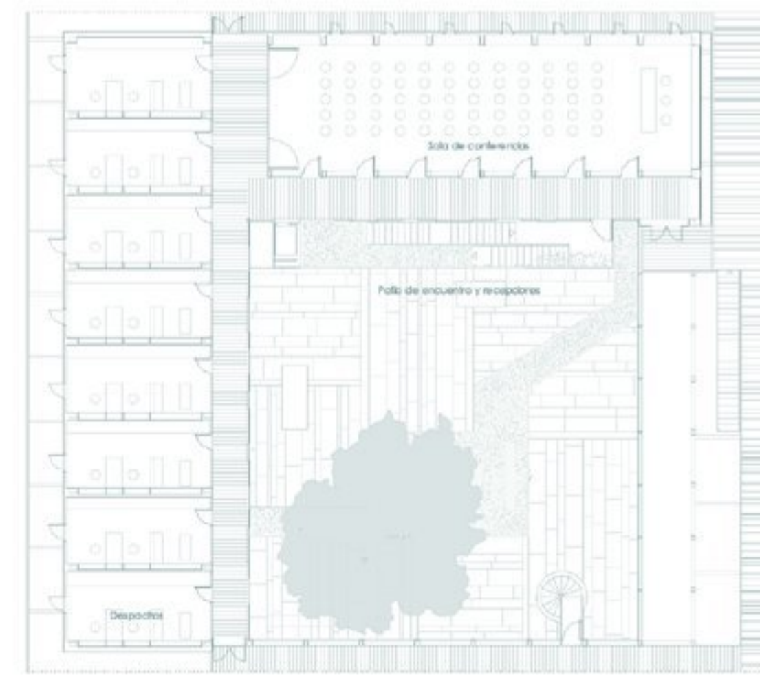
E09 PLANTA PRIMERA, ZONAS DE TRABAJO 1/200
