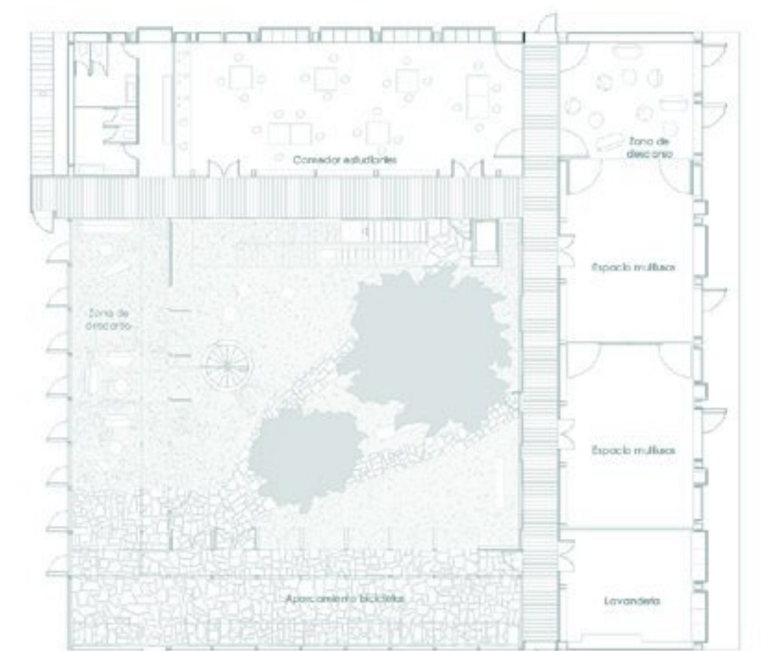
E16 PLANTA BAJA, ZONAS COMUNES 1/200
