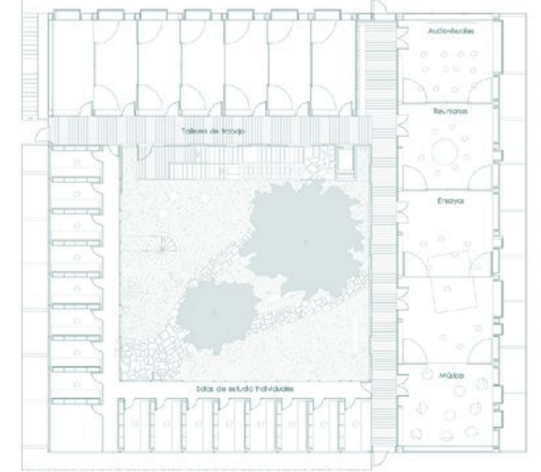
E11 PLANTA PRIMERA, ZONAS DE TRABAJO 1/200
