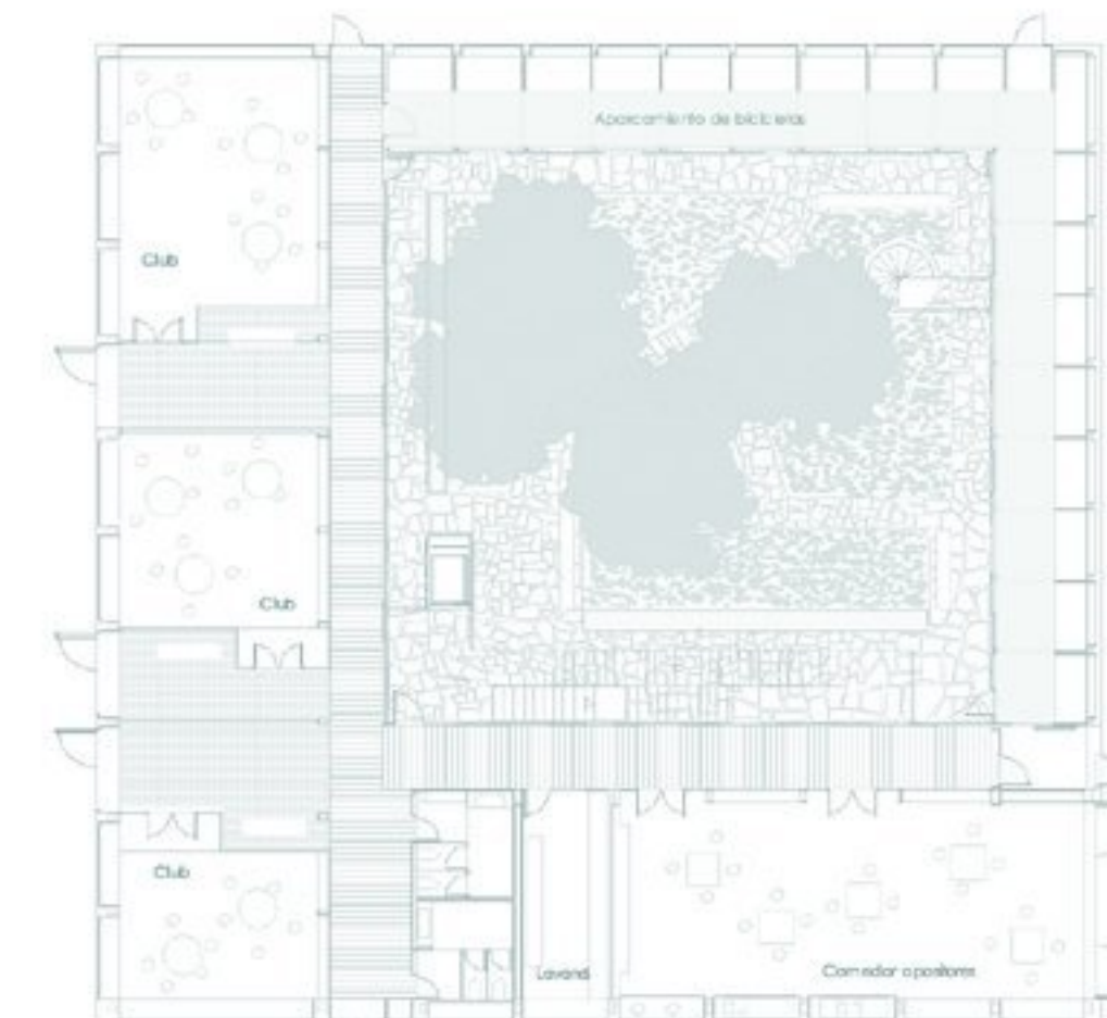
E15 PLANTA BAJA, ZONAS COMUNES 1/200
