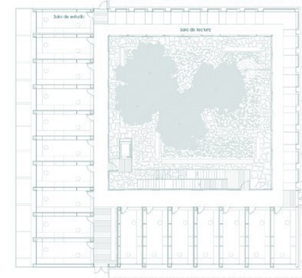
E10 PLANTA PRIMERA, ZONAS DE TRABAJO 1/200
