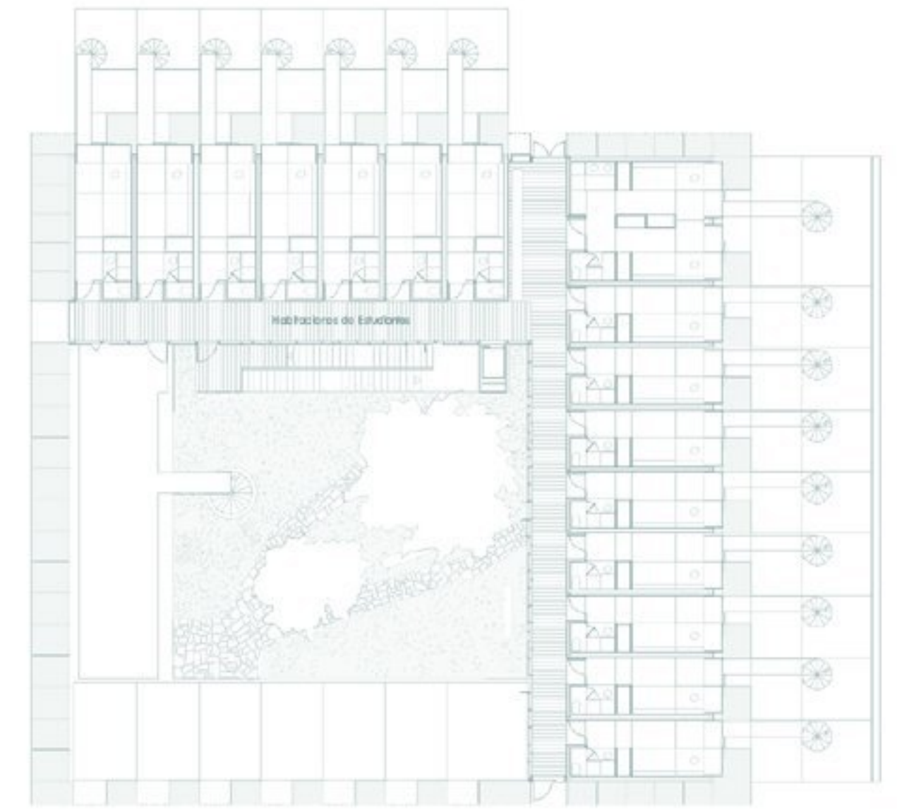
E06 PLANTA SEGUNDA/TERCERA, HABITACIONES 1/200
