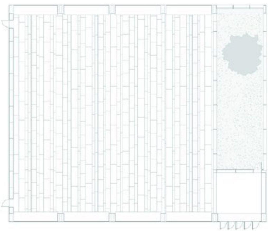
E12 PLANTA SALA DE EXPOSICIONES 1/200
