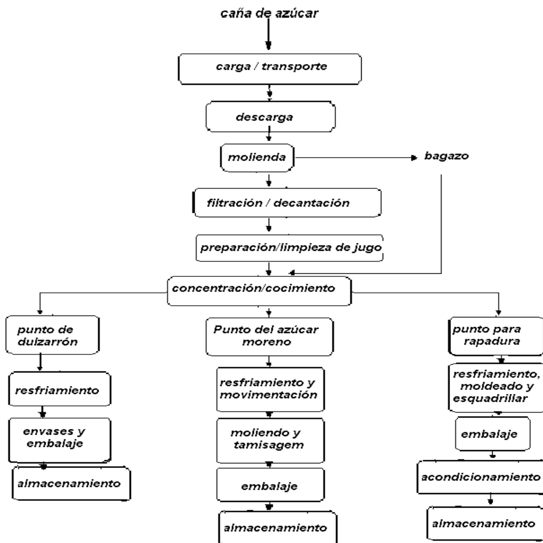
Figura 1. Flujograma de fabricación de los productos azucarados de la caña (adaptación de Silva et al. , 2003)
