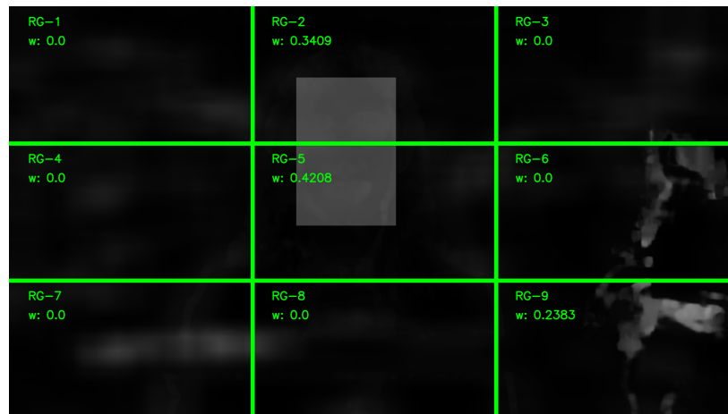
Figura C.15: Mapa de saliencia espacio-temporal con método SR y 50%-50%. Tres regiones.
