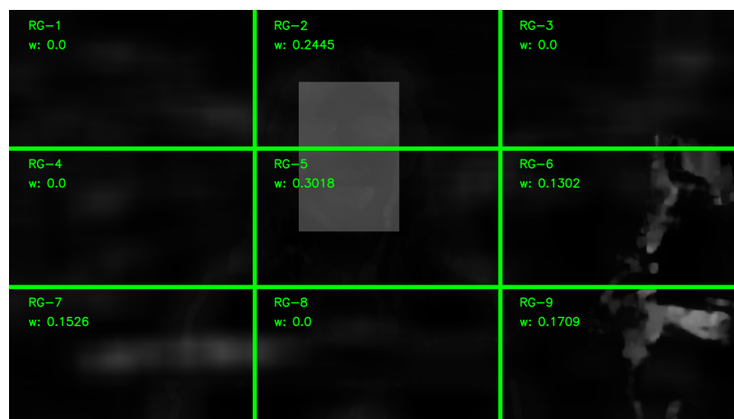
Figura C.17: Mapa de saliencia espacio-temporal con método SR y 50%-50%. Cinco regiones.
