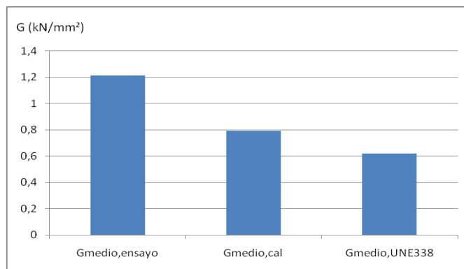
Figura 1. Valor del módulo de elasticidad transversal ( G_{medio} ) obtenido en el ensayo mecánico, calculado según EN 384:2010 y el correspondiente a la clase D24 de la norma EN 338:2010.
