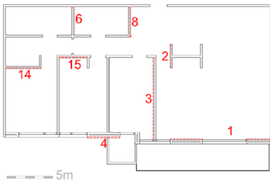
Figura 2: Planta de las viviendas.
