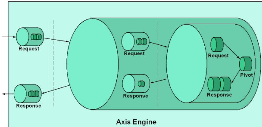
Figura 10 Esquema del motor de Axis
