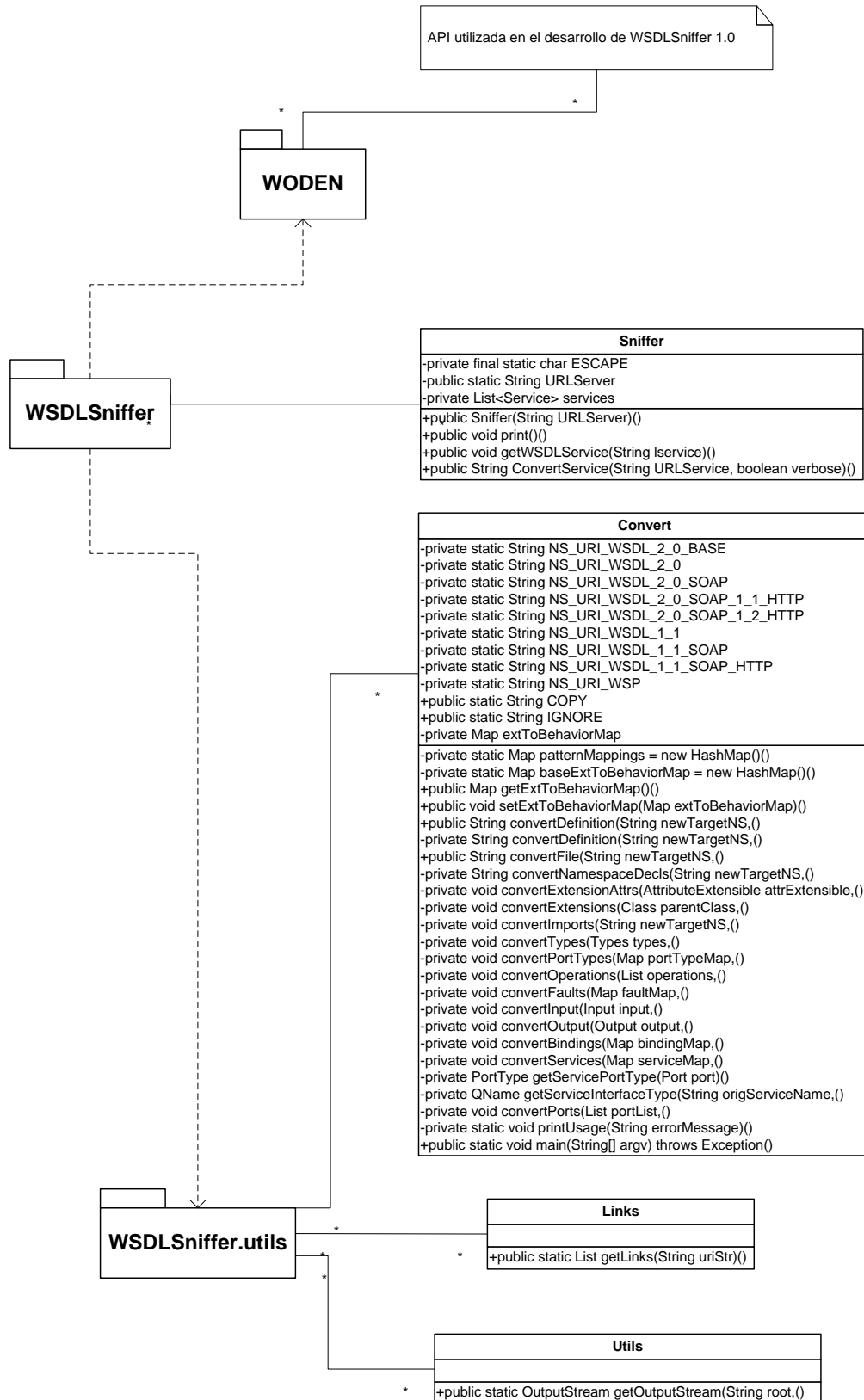
Figura 19 Clases utilizadas por WSDLSniffer
