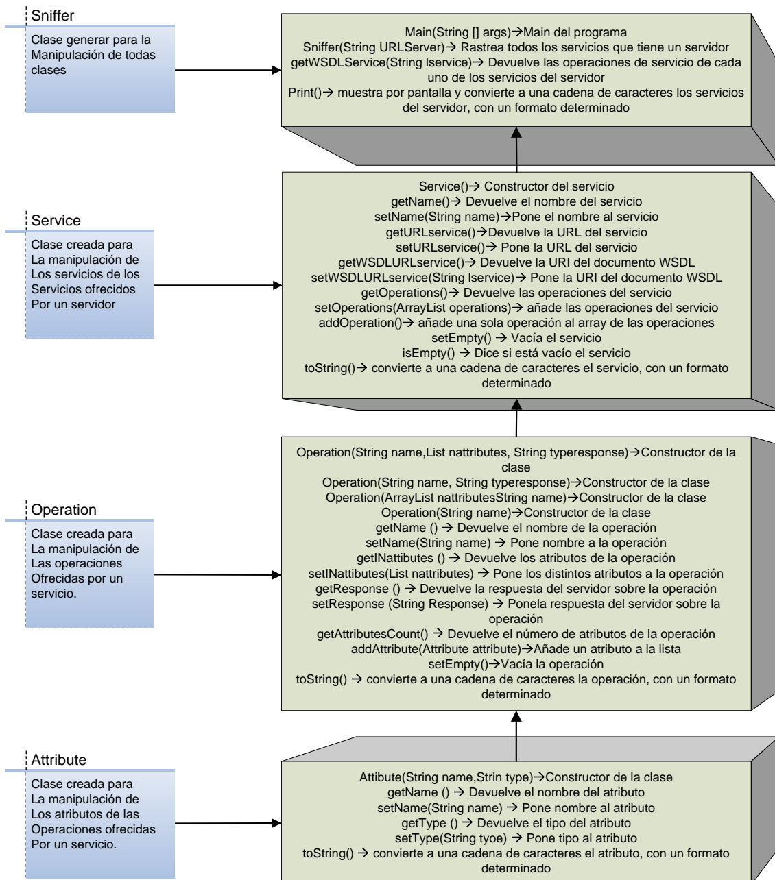
Figura 14 Esquema API WSDLSniffer
