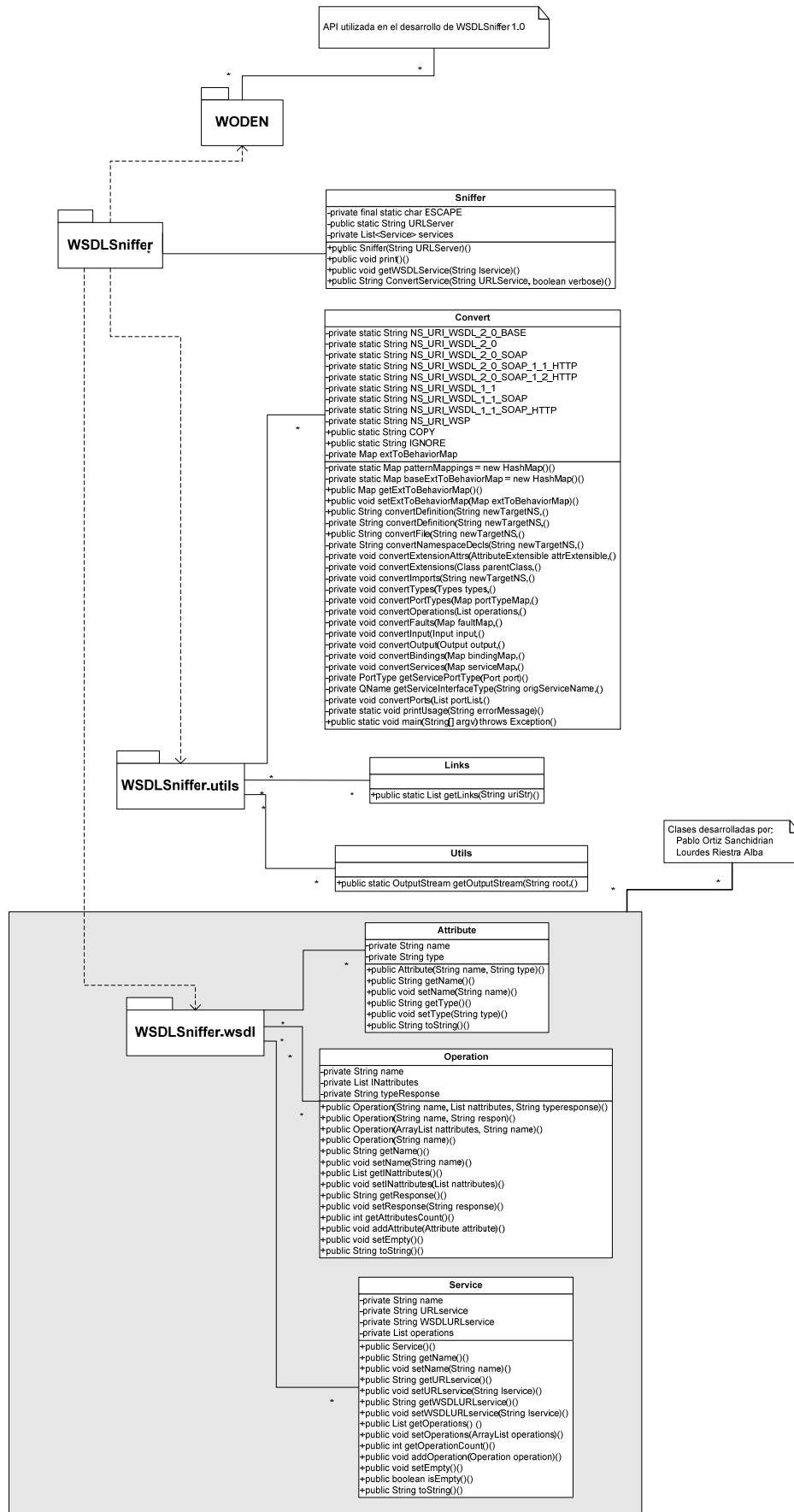
Figura 18 Diagrama general de clases WSDLSniffer 1.0
