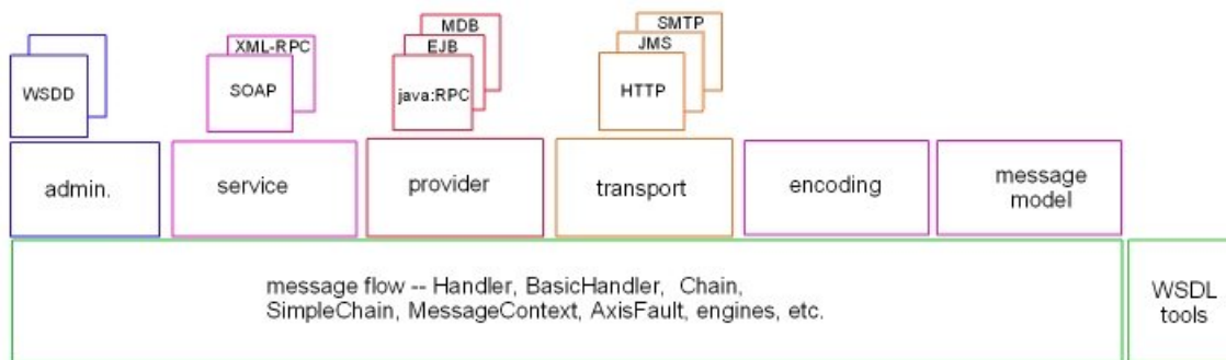
Figura 11 Sistema de capas y sub-sistemas de Axis
