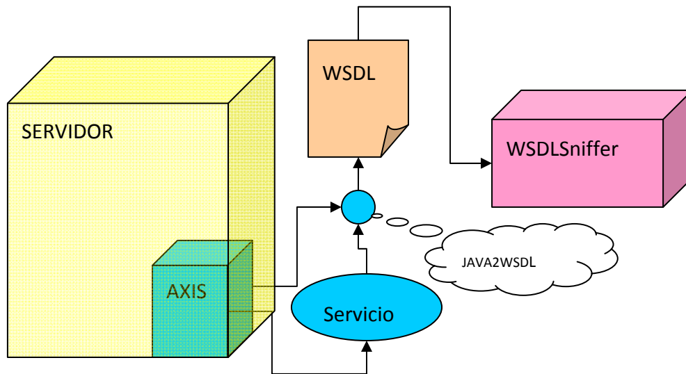
Figura 12 Esquema de dependencia de Axis
