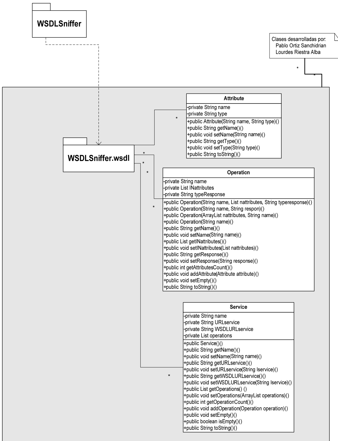
Figura 20 Clases desarrolladas para WSDLSniffer
