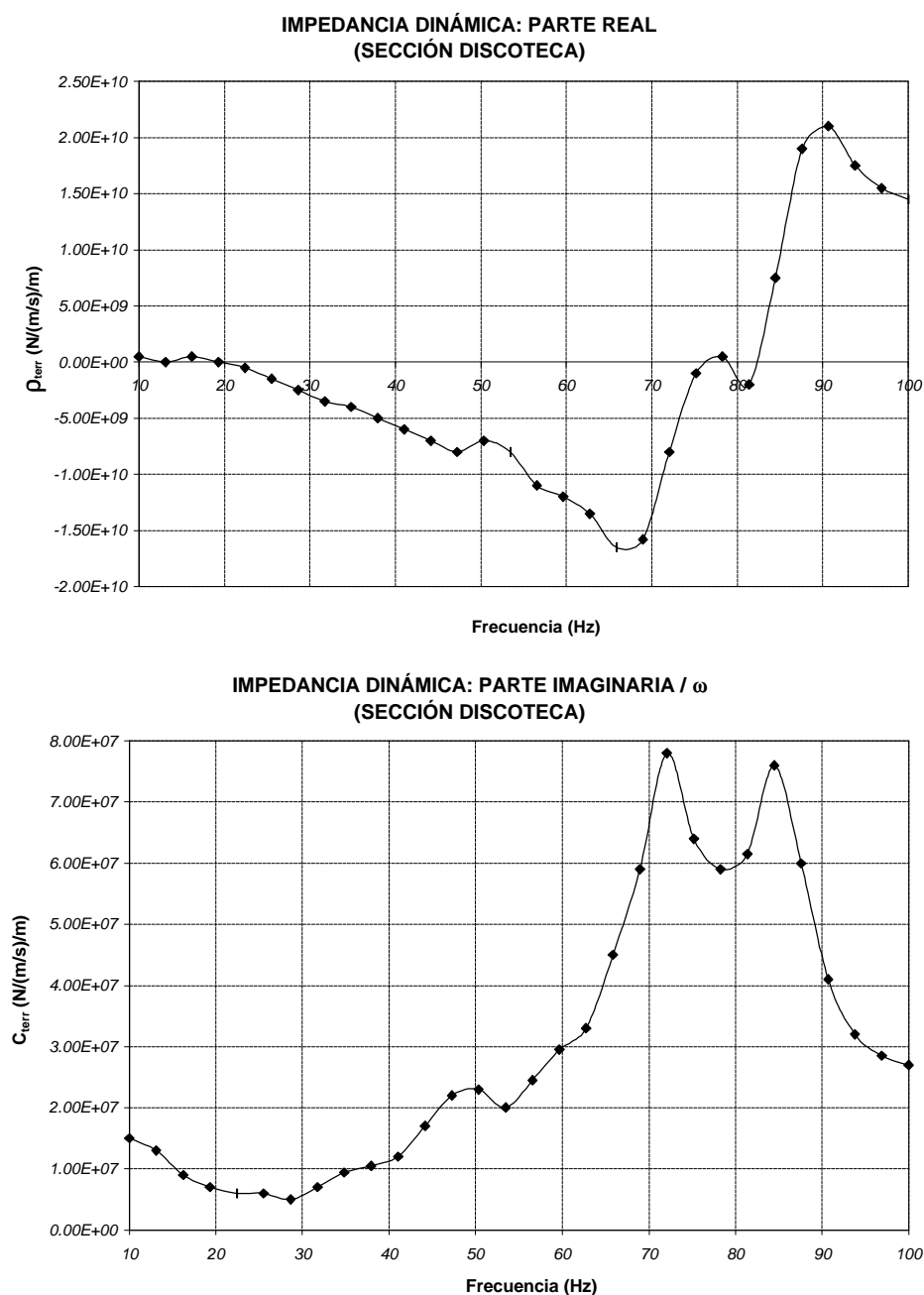
Figura 13: Impedancia dinámica de terreno y sostenimiento
