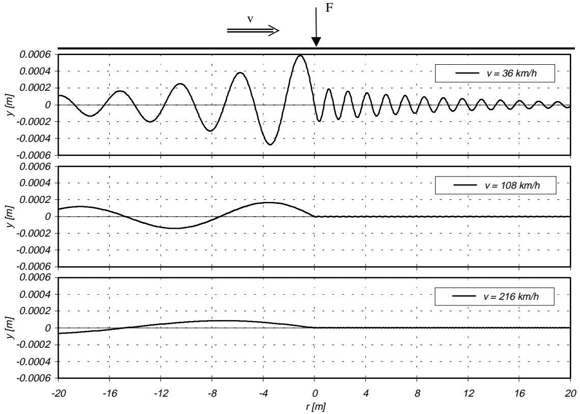
Figura 4: Desplazamientos en un sistema de coordenadas móvil con la carga
