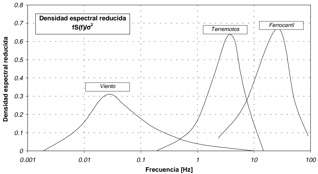
Figura 5: Densidades espectrales comparadas
