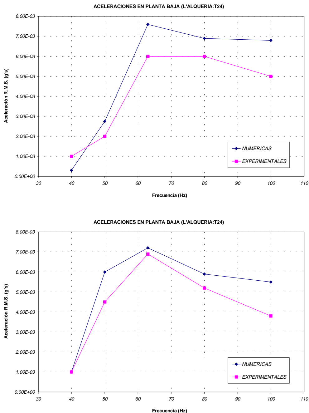
Figura 7: Resultados experimentales y ajuste del modelo
