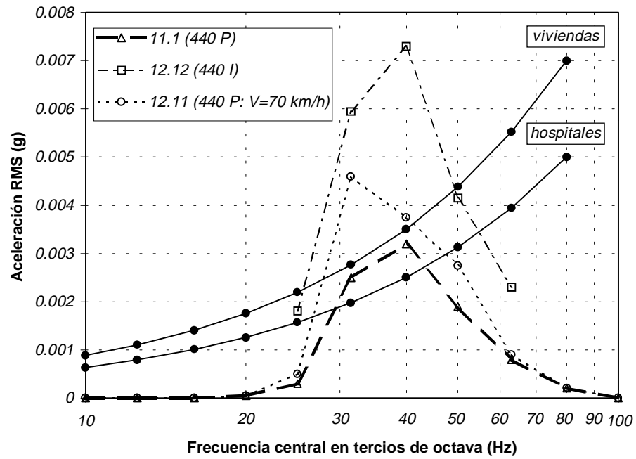
Figura 2: Efectos medidos y límites admisibles
