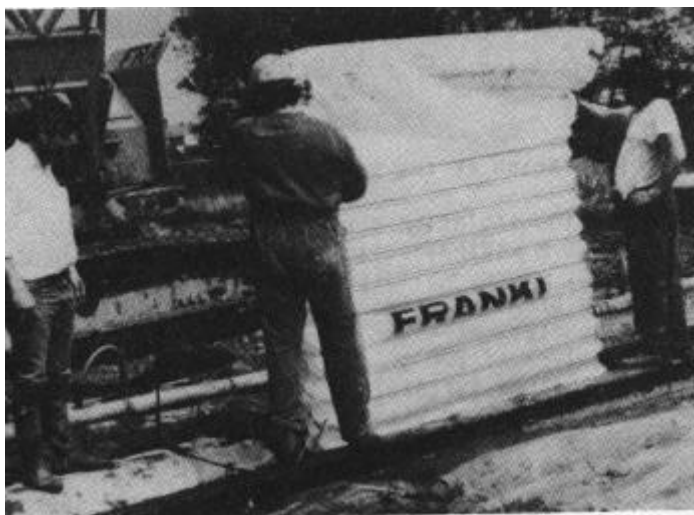
Figura 10: Sistema de construcción de una trinchera
