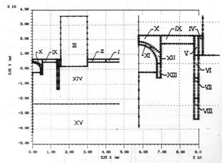
Figura 8: Malla con pantalla
