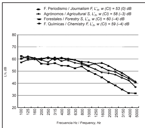
Figura 2. Nivel de presión sonora de impactos normalizado L'_n en los recintos objeto de ensayo. Figure 2. Normalized impact sound pressure level L'_n in the rooms tested.
