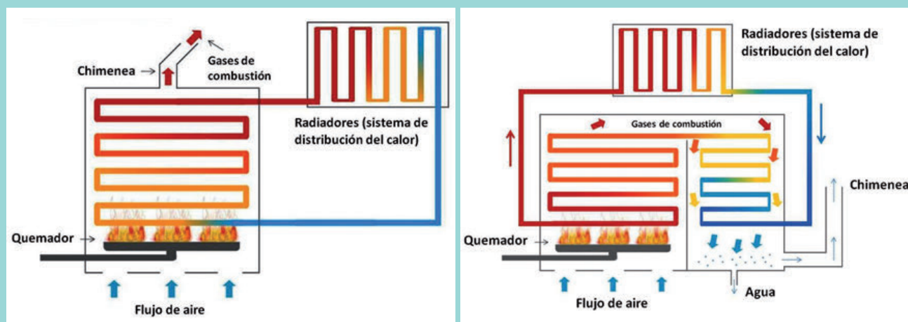
Figura 6. Esquemas de funcionamiento de una caldera convencional (izquierda) y de una caldera de condensación (derecha). El agua de color rojo, naranja o azul indica que está de mayor a menor temperatura, respectivamente.
