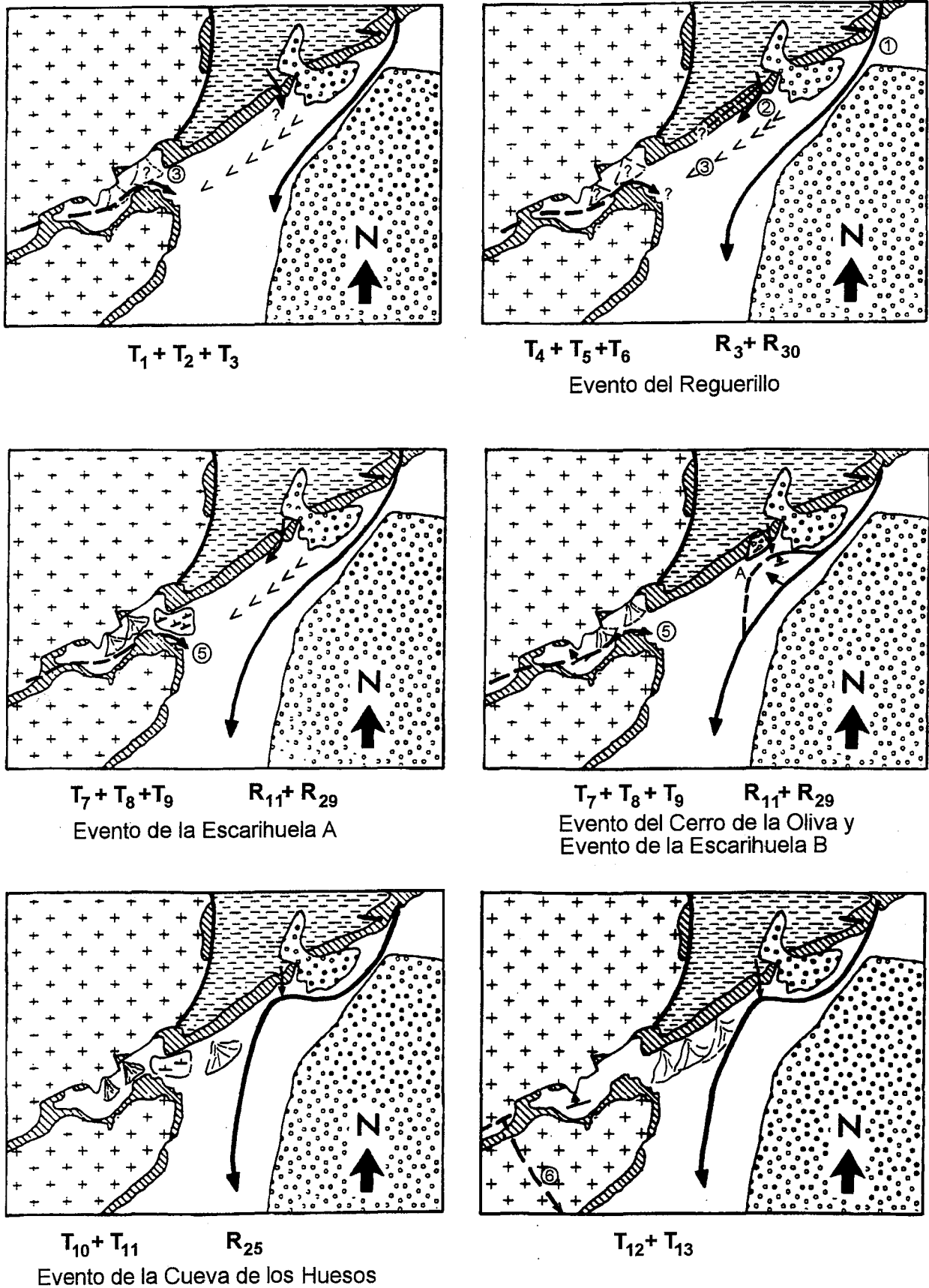
Fig. 2.- Evolución del sistema de los ríos Jarama-Lozoya-Guadalix y arroyo Miraflores durante el Plioceno terminal y Pleistoceno. 1- río Jarama, 2- río Lozoya, 3- abanicos aluviales de Redueña, 4- umbral, 5- arroyo Miraflores, 6- río Guadalix.
