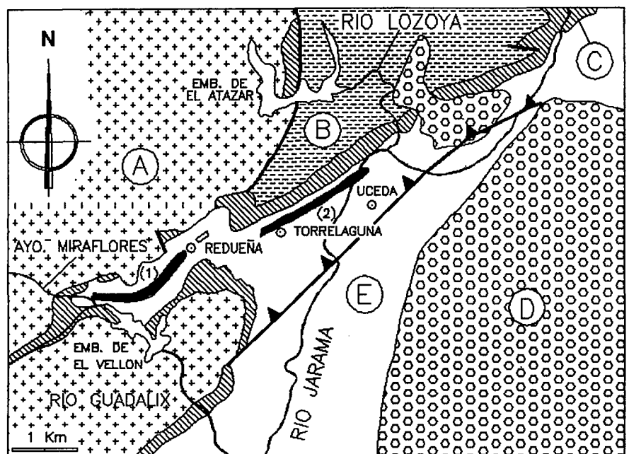
Fig. 1.- Situación geográfica y geológica de la zona de estudio. (1) Fosa de Redueña, (2) Fosa de Torrelaguna. A- Granito, B- Paleozoico, C- Mesozoico, D- Raña, E- Cuaternario.
