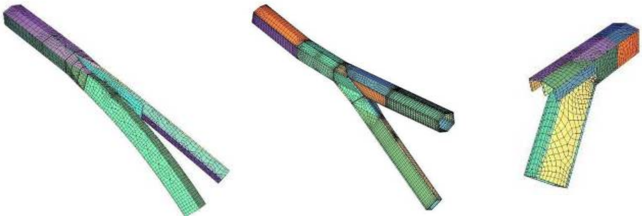
Fig.5 Vista de los modelos de cálculo empleados para el cálculo de dos de los nudos de unión entre patas y cordón superior realizados con el programa SOFISTK.
