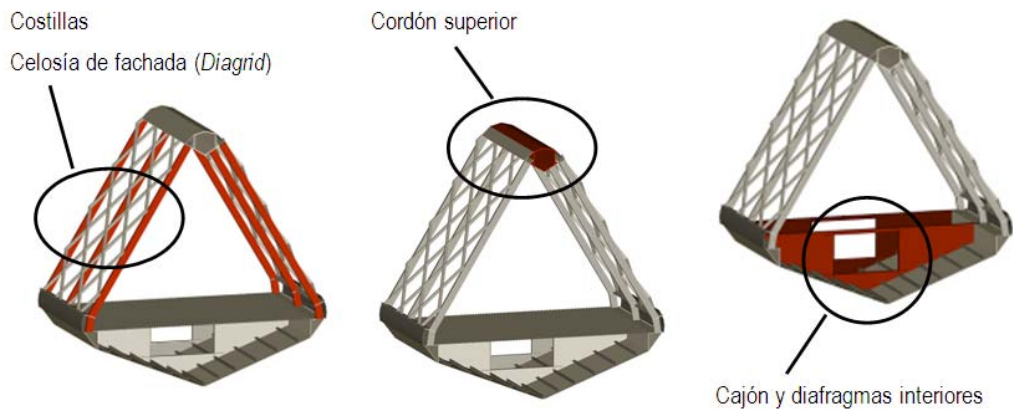
Fig. 3 Elementos estructurales principales
