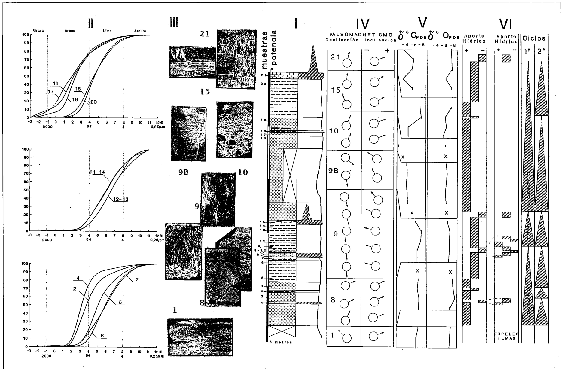
Fig. 2.— Estratigrafía (I), Granulometrías (II), Lámina transparente (III), Paleomagnetismo (IV), Isotopía (V), Interpretación paleoambiental (VI). (1) grava, (2) arena, (3) lutita, (4) espeleotema.
