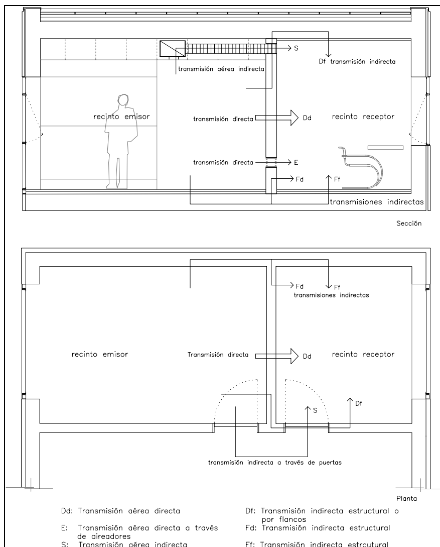
Figura 1. Definición de los caminos de transmisión del sonido entre dos recintos.
