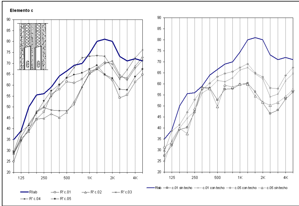
Figura 5. (Izquierda) Diferencia entre R' y R para el elemento c. (Derecha) Caso c, aislamiento acústico de recintos, con techo y sin techo suspendido.
