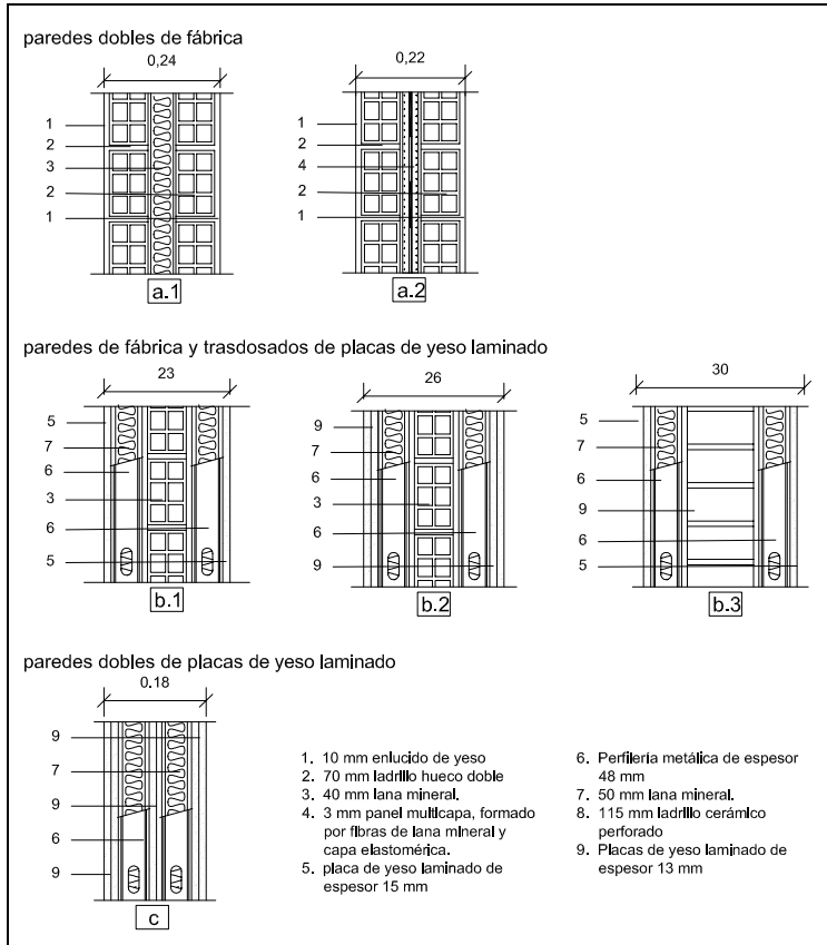
Figura 2. Elementos ensayados
