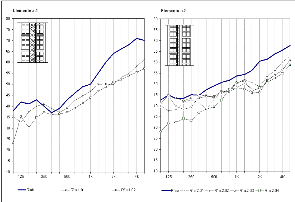
Figura 3. Diferencias entre R' y R para los elementos a.1 y a.2 respectivamente.
