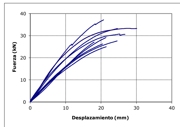
Fig. 3. Gráfico carga-desplazamiento de vigas planas.
