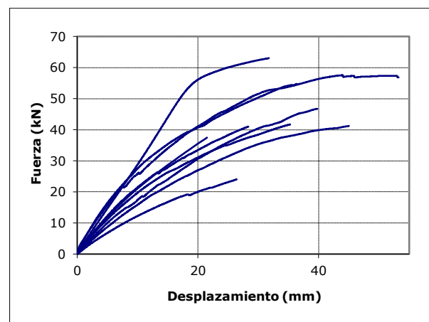
Fig. 4. Gráfico carga-desplazamiento de vigas de canto.
