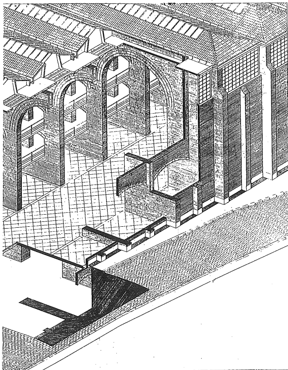
R. Monco: Museo de Mérida. Axonometría con el espacio interior pseudorromano y planta.
