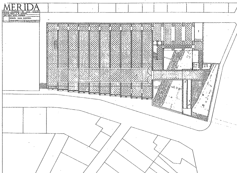
R. Monco: Museo de Mérida. Axonometría con el espacio interior pseudorromano y planta.
