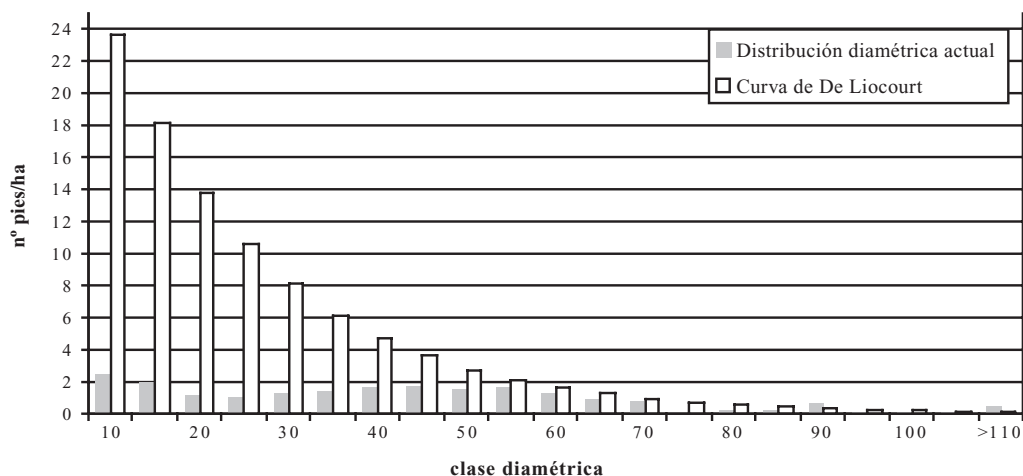
Figura 2. Distribución de clases diamétricas actual en la Dehesa de Candalija y distribución diámetro según la curva de Liocourt (Eq. 3)
