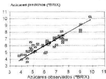
Figura 1. Comparación de los datos de azúcares (sólidos y solubles) observados y predichos a través del modelo espectral. Error del modelo \pm 0.69^\circ BRIX. El modelo ha sido validado en las I Jornadas de I. + D de la Universidad Politécnica de Madrid, por lo que se encuentra en proceso de solicitud de patente.
