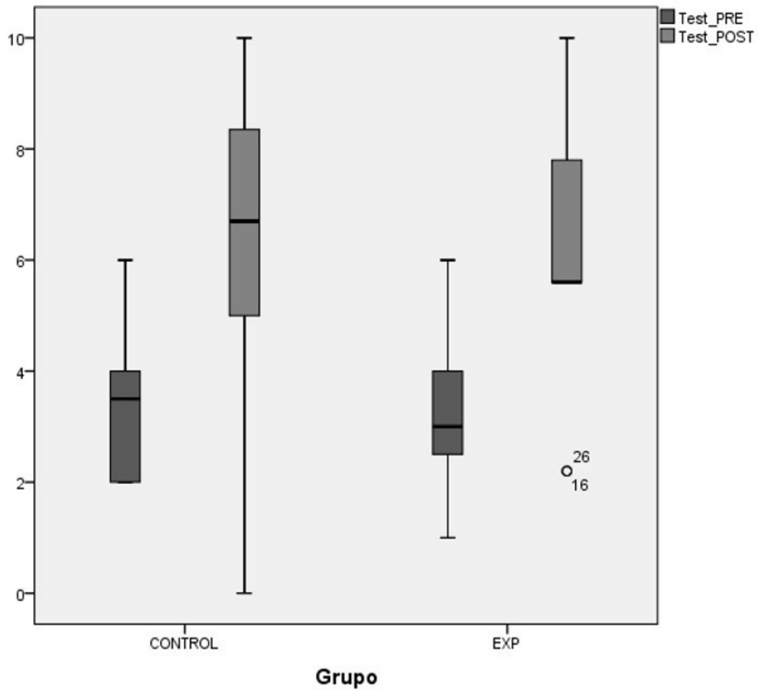
Figura 1. Diagrama de cajas de las puntuaciones del test de competencia matemática en estadística para los dos grupos de estudios antes (Test_PRE) y después (Test_POST) de la intervención. EXP: Grupo PEDAL.
