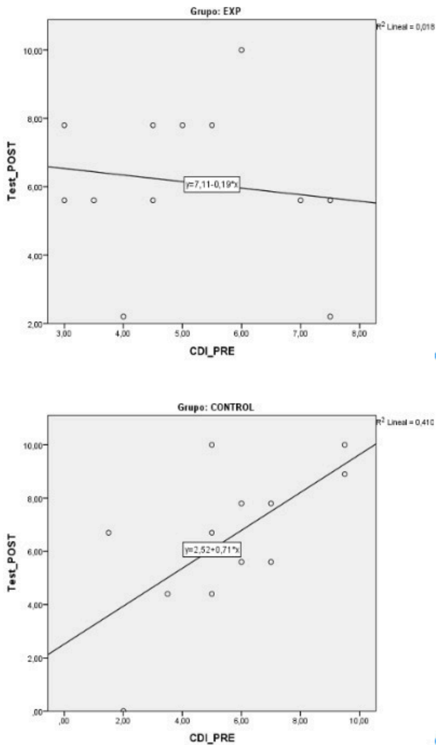
Figura 2. Correlación y ajuste lineal entre el nivel previo a la intervención en estadística (CDI_PRE) y la puntuación del test de competencia matemática en estadística tras la intervención (Test_POST) para los dos grupos de estudio. EXP: Grupo PEDAL.
