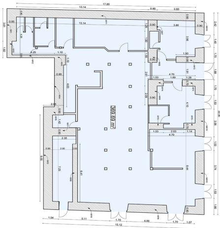
PLANTA
