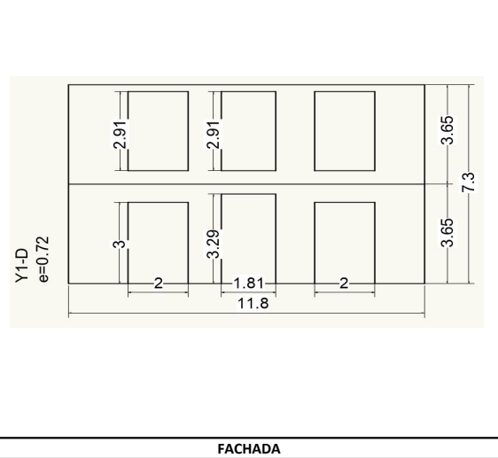
FACHADA
