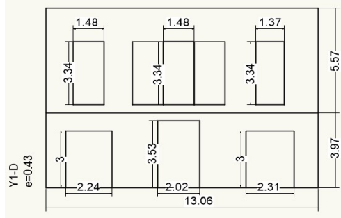
FACHADA
