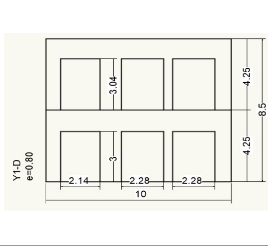
FACHADA
