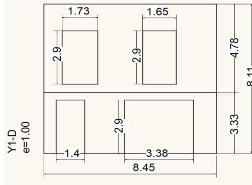
FACHADA
