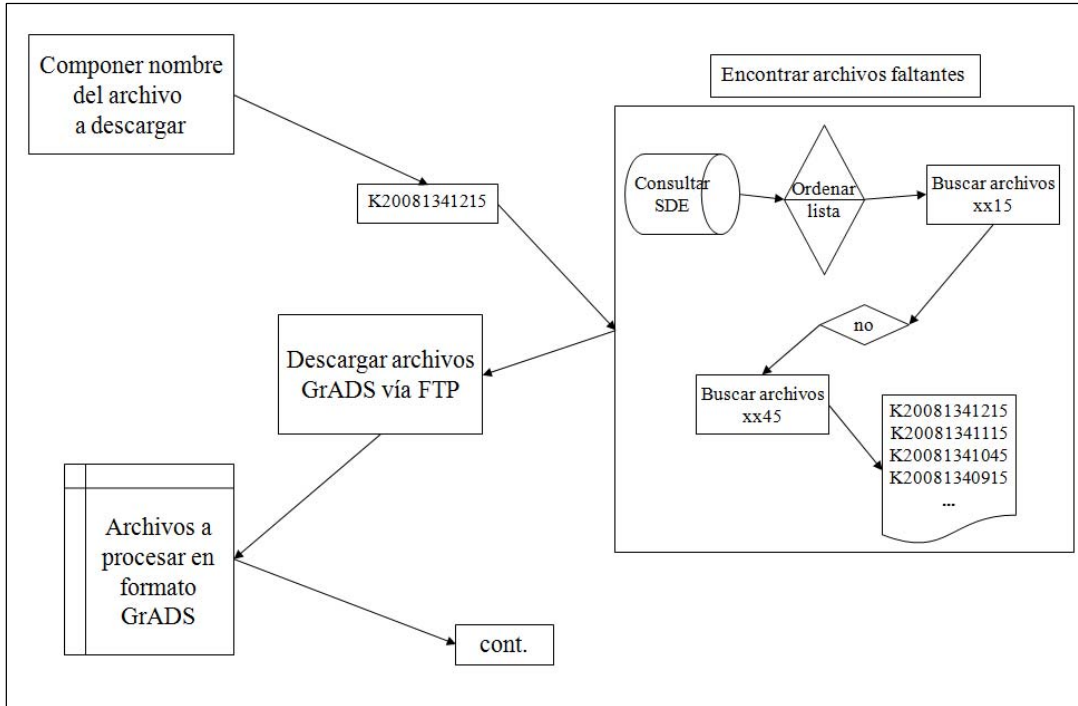
Fig 1. Aplicación del servidor. Modelo de procesos
