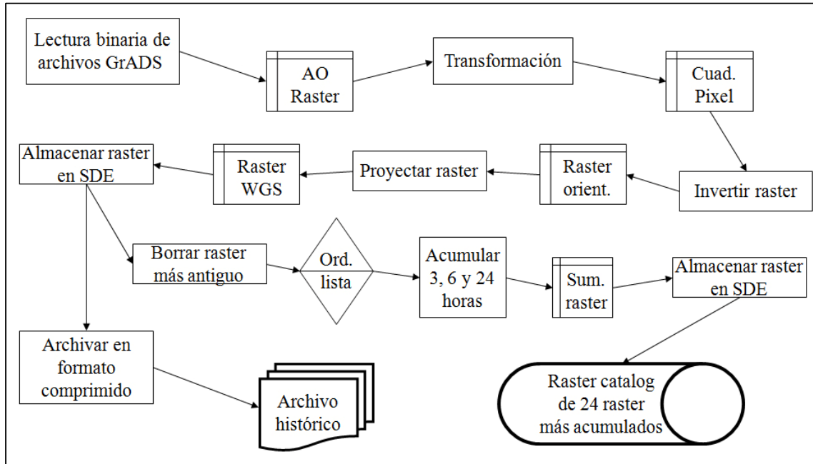
Fig 2. Aplicación del servidor. Modelo de procesos
