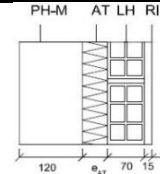
Figura 56. F12.E.0 sin cámara de aire
