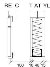
Figura 52. F10.I.3 con cámara de aire ventilada
