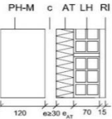
Figura 57. F12.E.0 con cámara de aire no ventilada
