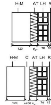
Figura 61. F13.G.0 sin cámara de aire
