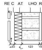
Figura 46. F8.C.3 con cámara de aire ventilada
