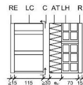
Figura 29. F5.A.1 sin cámara de aire
