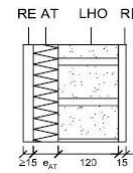
Figura 26. F4.C.1 sin cámara de aire
