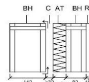
Figura 12. F2.B.0 con cámara de aire ventilada
