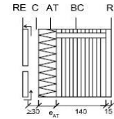
Figura 47. F8.D.3 con cámara de aire ventilada
