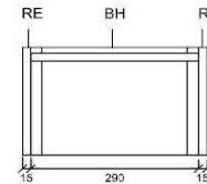
Figura 49. F9.B.1 con cámara de aire ventilada
