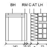
Figura 7. F1.B.0 con cámara de aire no ventilada
