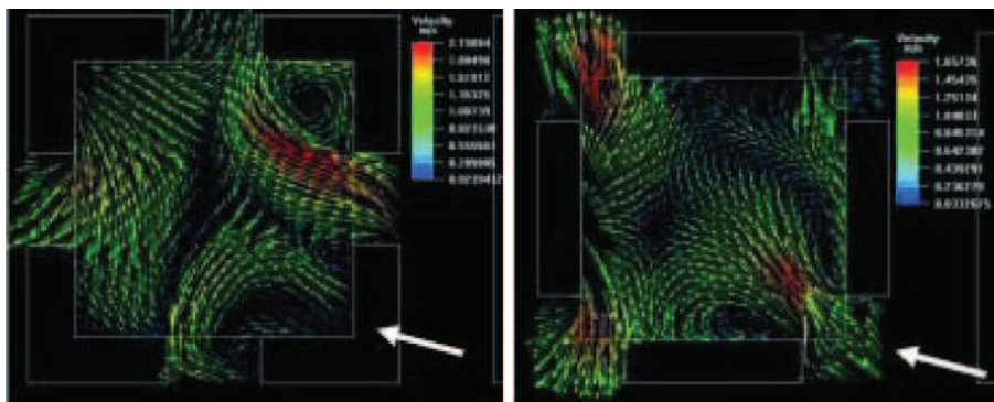
Figura 16. Resultados de la simulación de viento para la plaza con distinta ubicación de aperturas. Queda reflejado el efecto negativo sobre la incidencia del viento por la apertura de la plaza en los extremos.
