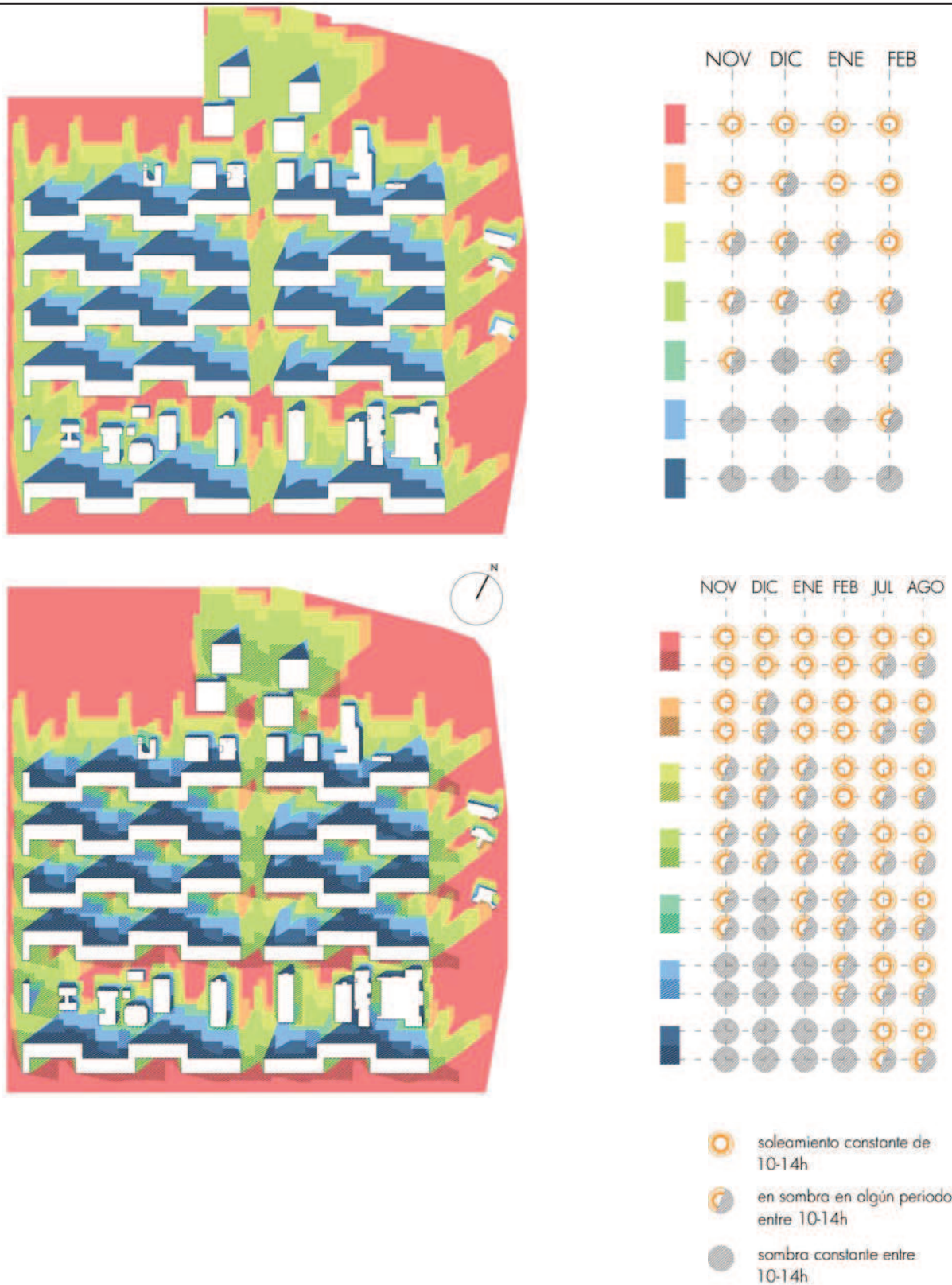
Fig. 22. Zonificación del espacio público según criterios de soleamiento en invierno (izq) y verano (derecha)
