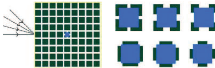
Figura 15. Representación gráfica del ejemplo analizado mediante programas de simulación CFD, con direcciones de viento 0°, 15°, 30° y 45°. La plaza analizada se encuentra rodeada por bloques de 18m de altura. A la derecha se puede ver las variaciones de tamaño y posición de aperturas que se ensayaron en el modelo.
