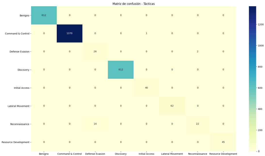
Figura 8.13: Matriz de confusión de la identificación de tácticas para el árbol de decisión
