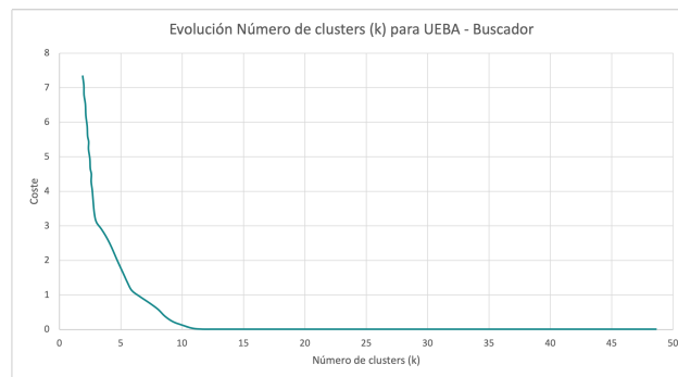
Figura 7.31: Coste - K-Means - Número de clusters - Buscador (UEBA)
