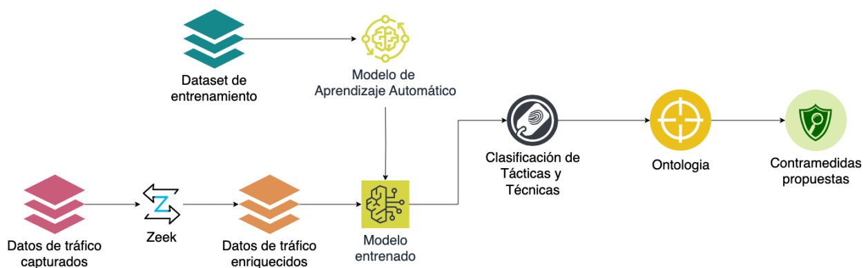
Figura 8.2: Metodología propuesta para la caracterización de TTPs
