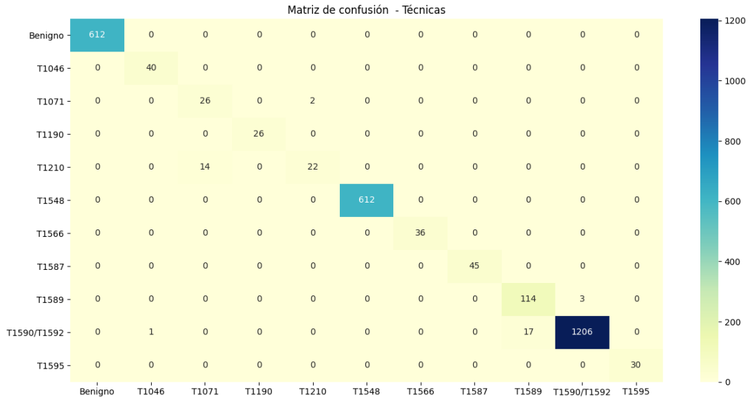
Figura 8.16: Matriz de confusión de la identificación de técnicas para Random Forest
