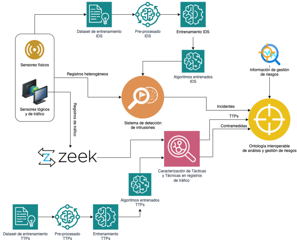
Figura 6.1: Arquitectura global del modelo propuesto
