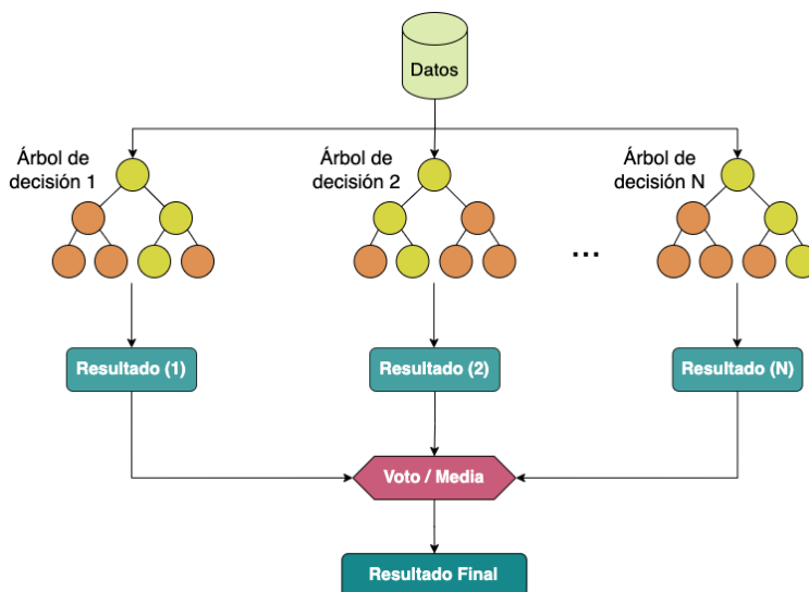
Figura 4.3: Esquema de funcionamiento del algoritmo Random Forest
