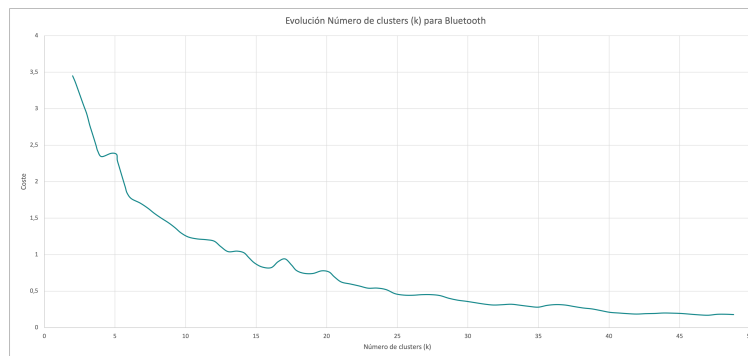
Figura 7.22: Coste - K-Means - Número de clusters - Bluetooth
