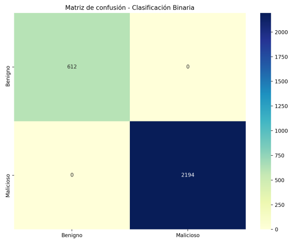
Figura 8.22: Matriz de confusión de la clasificación binaria para XGBoost
