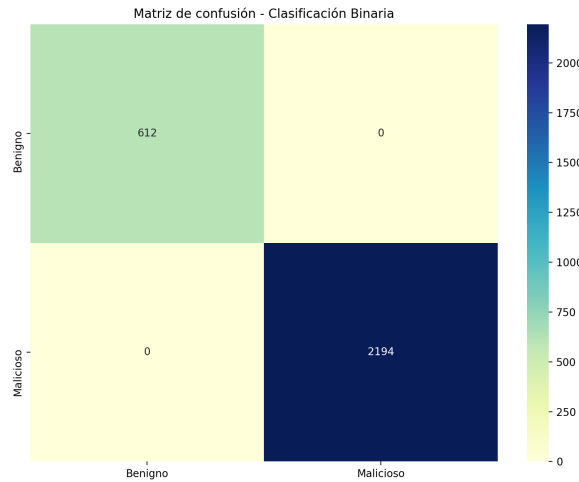
Figura 8.14: Matriz de confusión de la clasificación binaria para el árbol de decisión
