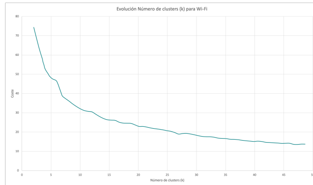
Figura 7.24: Coste - K-Means - Número de clusters - Wi-Fi
