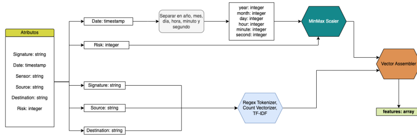
Figura 7.10: Pre-procesado de datos de SIEM
