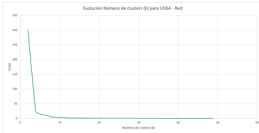
Figura 7.35: Coste - K-Means - Número de clusters - Red (UEBA)
