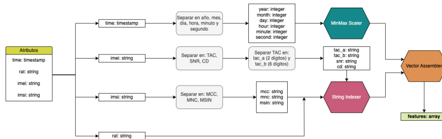
Figura 7.5: Pre-procesado de datos de sensor de redes móviles
