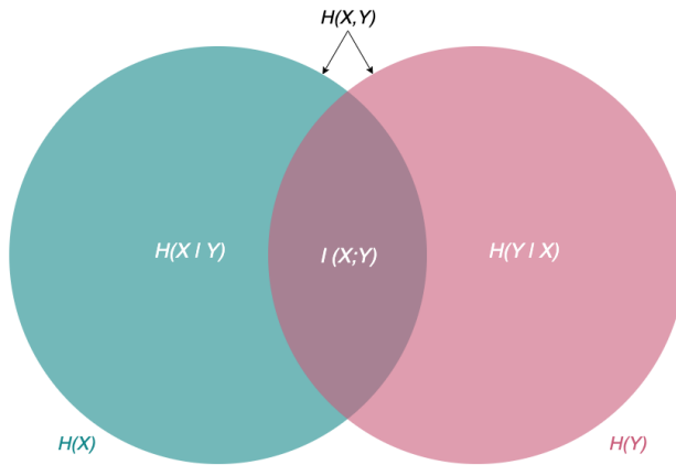
Figura 4.5: Diagrama de Venn sobre la relación entre información mutua y entropía
