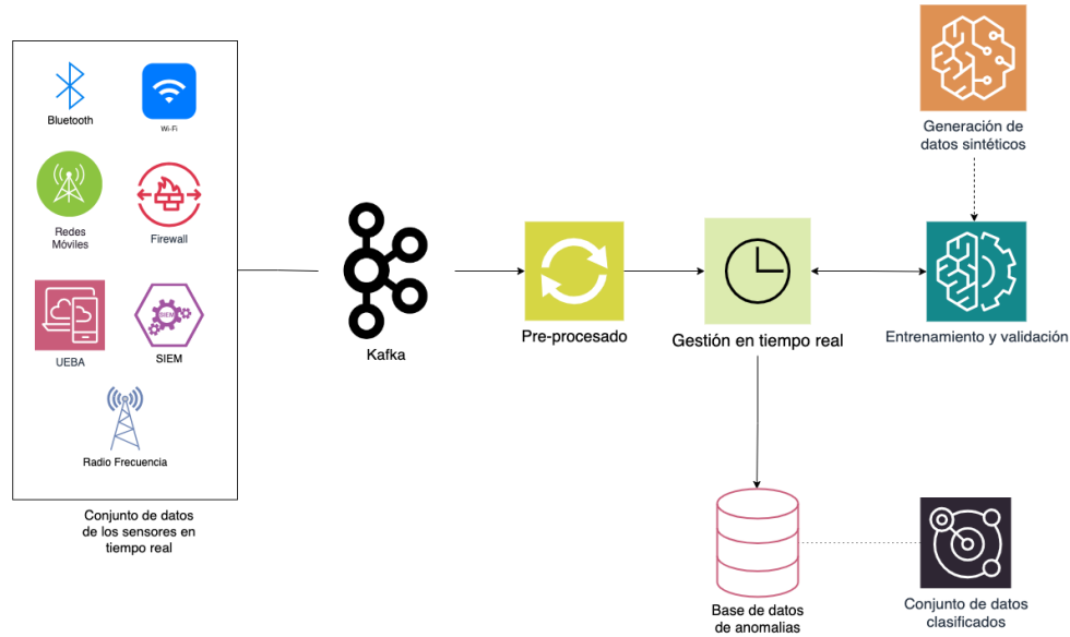
Figura 7.2: Arquitectura de la propuesta
