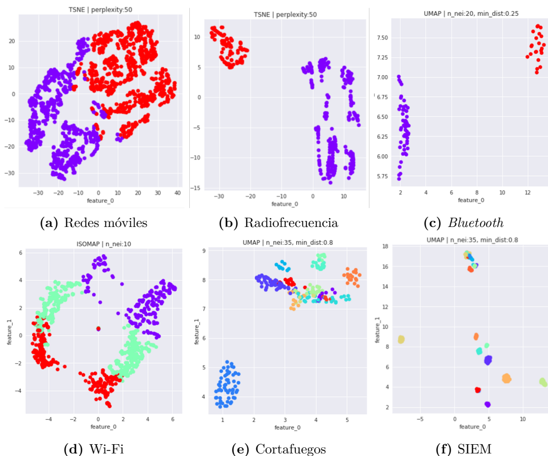
Figura 7.48: Representación de los clusters de cada fuente
