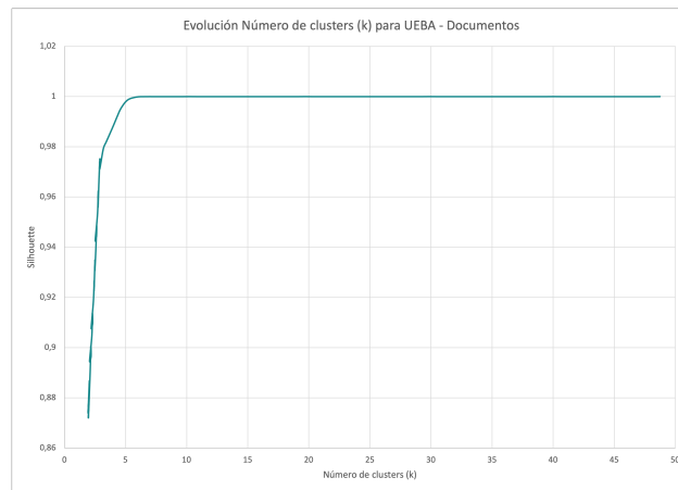
Figura 7.33: Métrica Silhouette - K-Means - Número de clusters - Documentos (UEBA)
