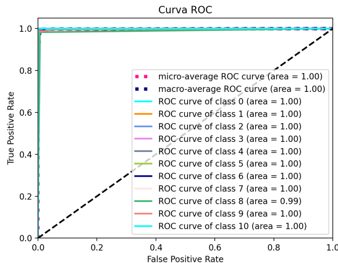
Figura 8.15: Curva ROC del modelo árbol de decisión
