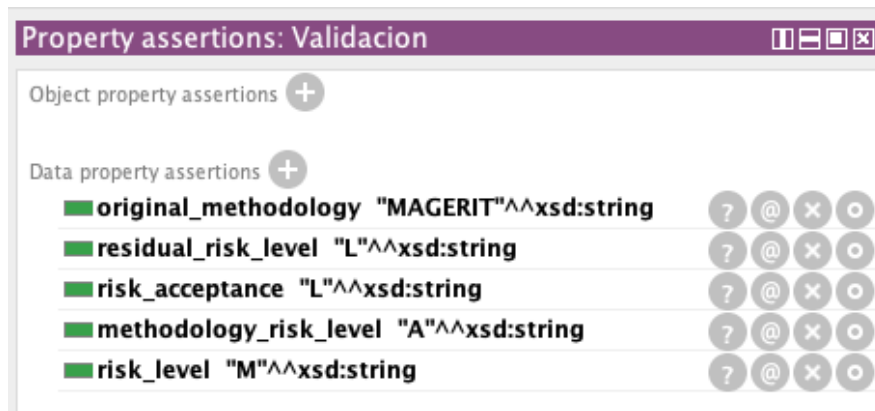
Figura 10.5: Nivel de riesgo residual global del sistema. Validación - Caso de uso 1.2
