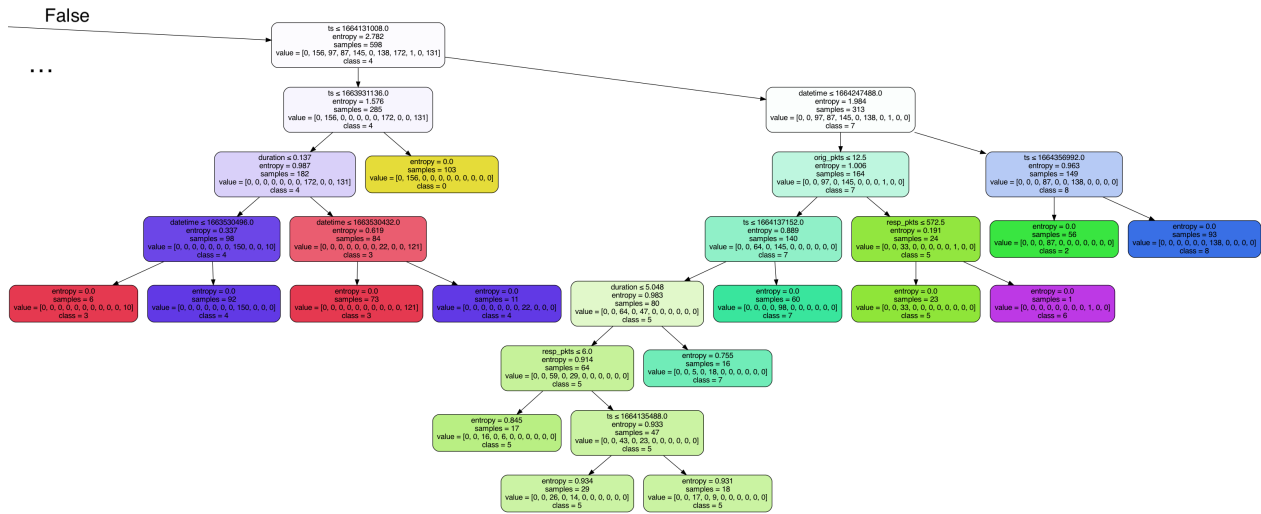
Figura 8.7: Estructura parcial de árbol del segundo estimador del modelo Random Forest
