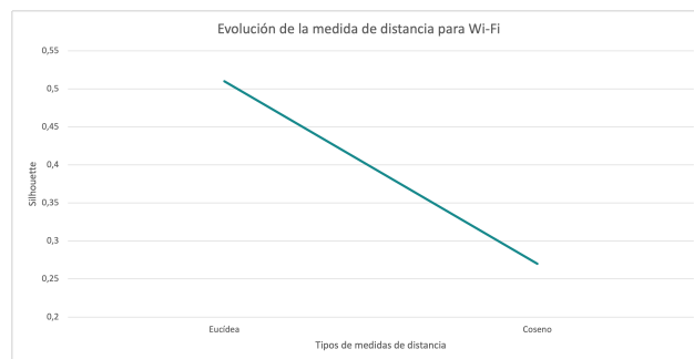
Figura 7.25: Métrica Silhouette - K-Means - Medida de la distancia - Wi-Fi
