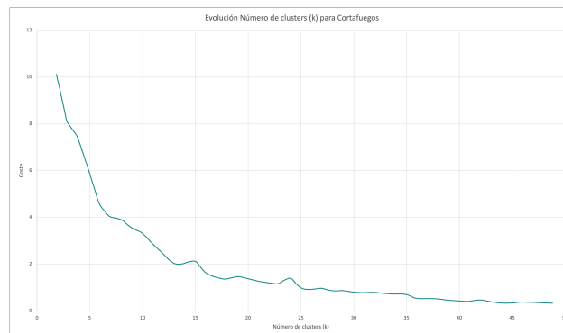
Figura 7.26: Coste - K-Means - Número de clusters - Cortafuegos
