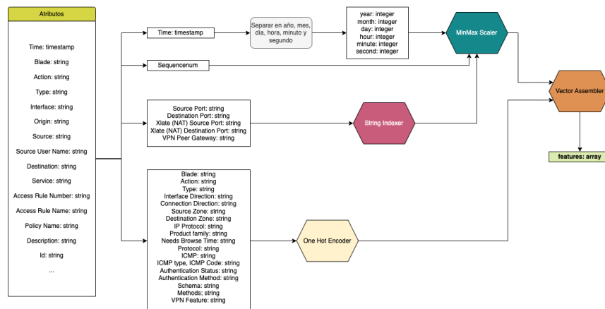
Figura 7.9: Pre-procesado de datos de cortafuegos
