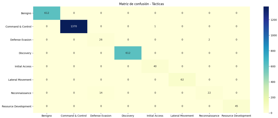
Figura 8.17: Matriz de confusión de la identificación de tácticas para Random Forest
