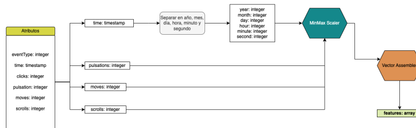
Figura 7.11: Pre-procesado de datos de actividad (UEBA)
