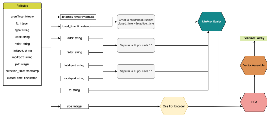
Figura 7.16: Pre-procesado de datos de sockets (UEBA)
