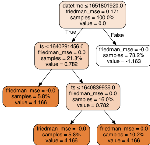
Figura 8.9: Estructura de árbol del primer estimador del modelo XGBoost
