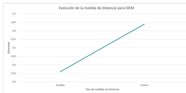
Figura 7.29: Métrica Silhouette - K-Means - Medida de la distancia - SIEM
