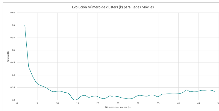
Figura 7.18: Métrica Silhouette - K-Means - Número de clusters - Redes móviles
