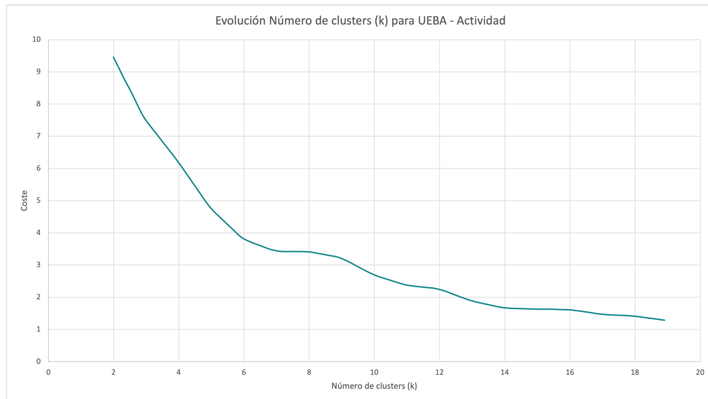
Figura 7.30: Coste - K-Means - Número de clusters - Actividad (UEBA)
