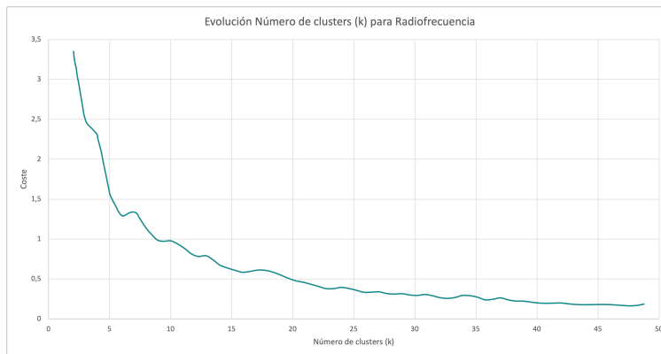
Figura 7.20: Coste - K-Means - Número de clusters - Radiofrecuencia
