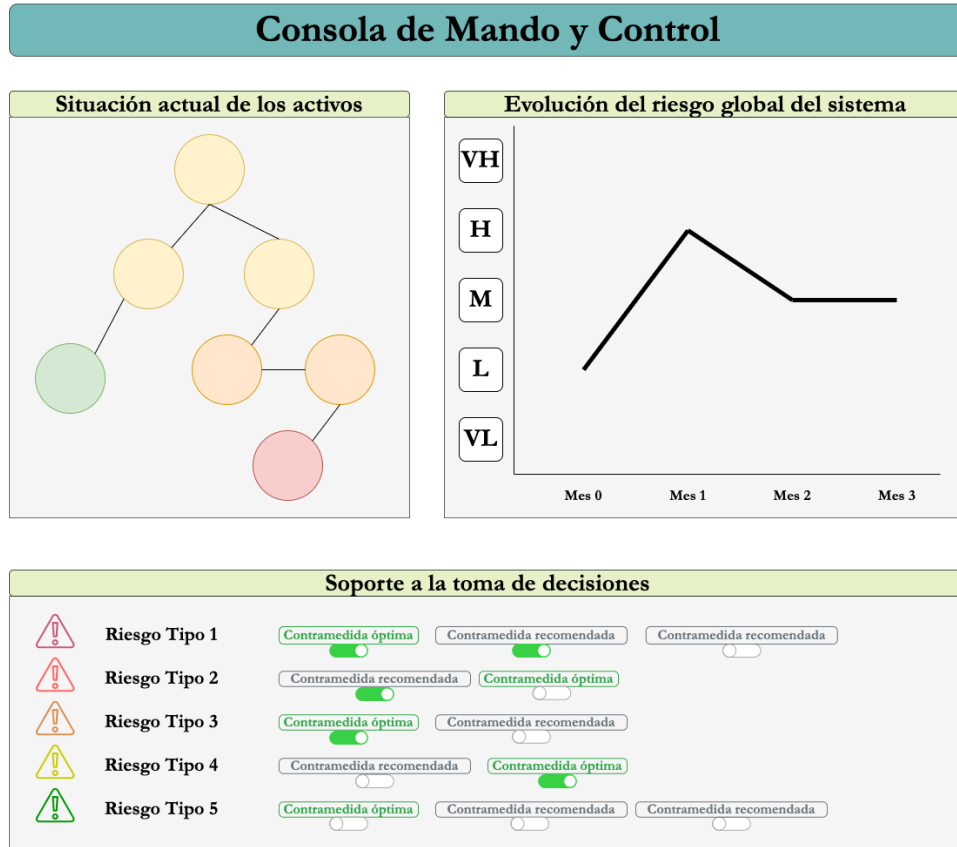
Figura 10.9: Prototipo de consola de mando y control
