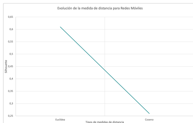
Figura 7.19: Métrica Silhouette - K-Means - Medida de la distancia - Redes móviles
