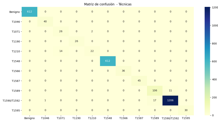
Figura 8.20: Matriz de confusión de la identificación de técnicas para XGBoost
