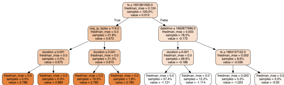
Figura 8.10: Estructura de árbol del segundo estimador del modelo XGBoost
