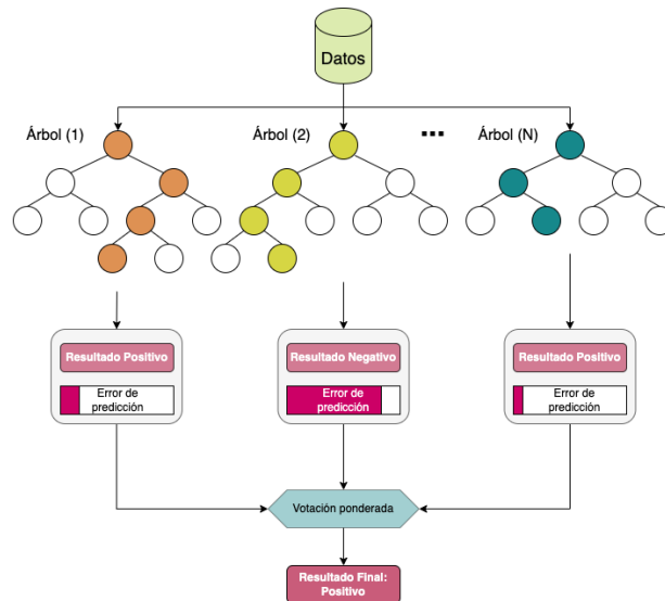
Figura 4.4: Esquema de funcionamiento del algoritmo XGBoost
