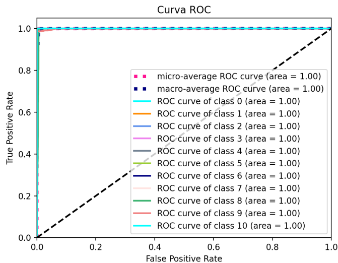
Figura 8.19: Curva ROC del modelo Random Forest
