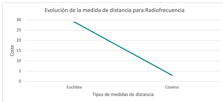
Figura 7.21: Coste - K-Means - Medida de la distancia - Radiofrecuencia
