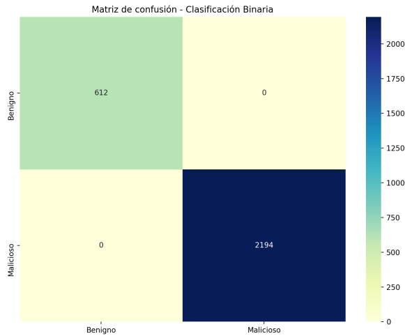
Figura 8.18: Matriz de confusión de la clasificación binaria para Random Forest
