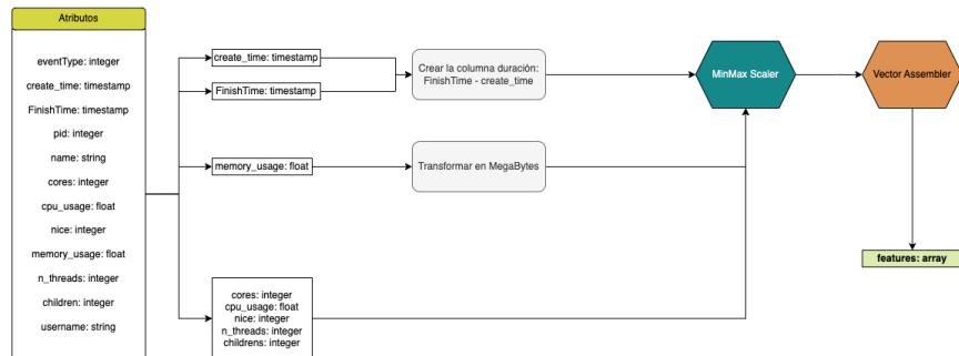
Figura 7.15: Pre-procesado de datos de procesos (UEBA)
