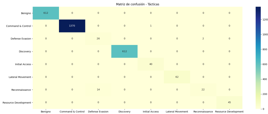
Figura 8.21: Matriz de confusión de la identificación de tácticas para XGBoost
