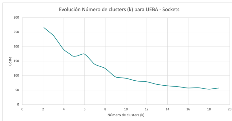
Figura 7.39: Coste - K-Means - Número de clusters - Sockets (UEBA)
