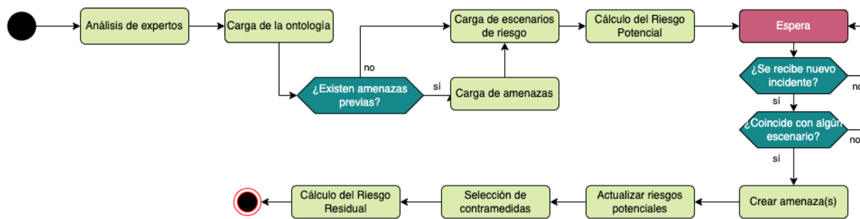
Figura 9.11: Flujo de trabajo del gestor de la ontología
