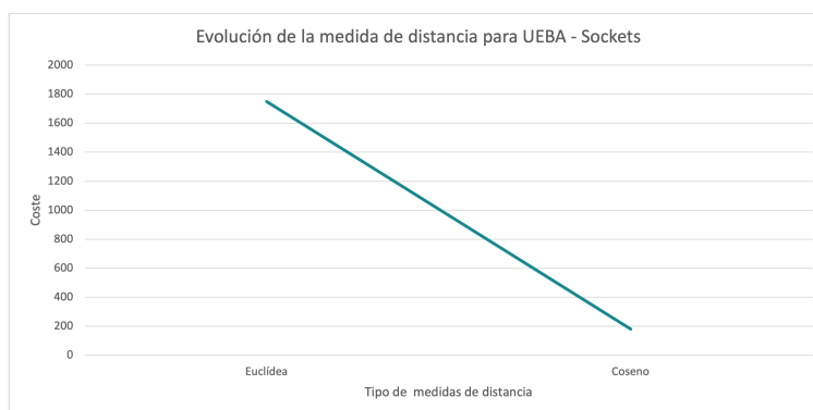
Figura 7.40: Coste - K-Means - Medida de la distancia - Sockets (UEBA)
