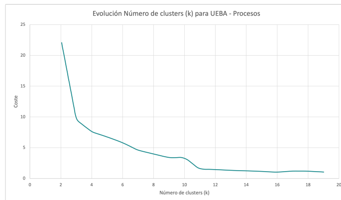
Figura 7.37: Coste - K-Means - Número de clusters - Procesos (UEBA)
