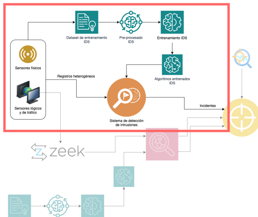
Figura 7.1: Módulo IDS en la arquitectura global propuesta
