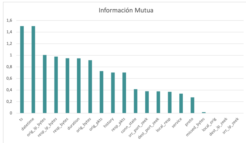
Figura 8.3: Información mutua de las columnas del dataset
