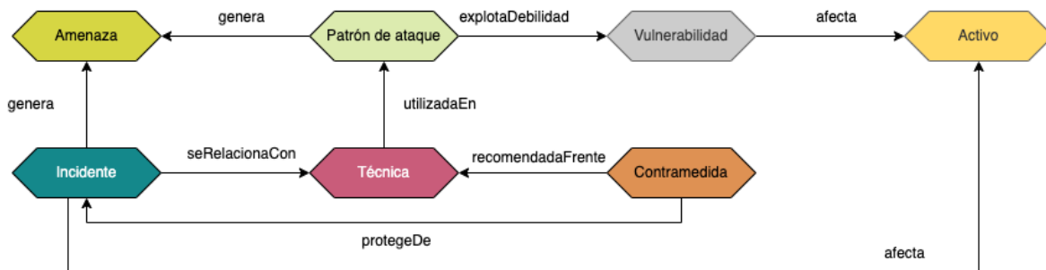
Figura 8.11: Ontología propuesta
