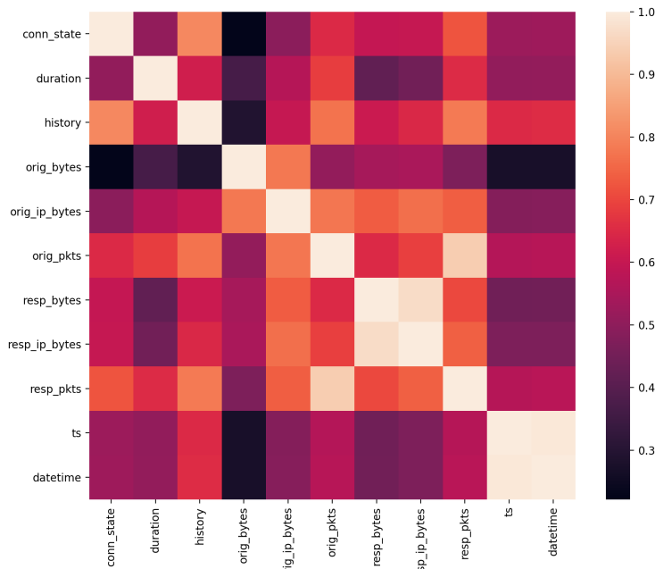
Figura 8.4: Matriz de correlación del conjunto UWF-ZeekDataFall22
