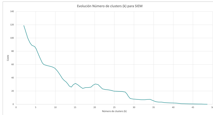
Figura 7.28: Coste - K-Means - Número de clusters - SIEM
