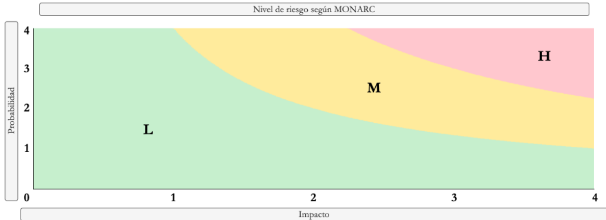
Figura 9.7: Mapa de calor para el cálculo del riesgo en MONARC
