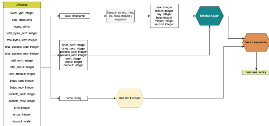
Figura 7.14: Pre-procesado de datos de red (UEBA)
