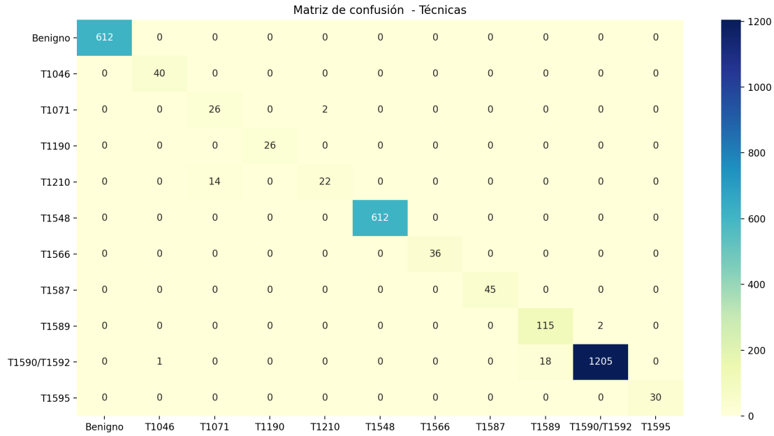
Figura 8.12: Matriz de confusión de la identificación de técnicas para el árbol de decisión
