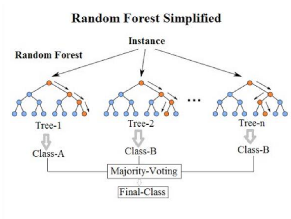
Figura 7. Ejemplo de Random Forest simplificado. Figura extraída de [18]
