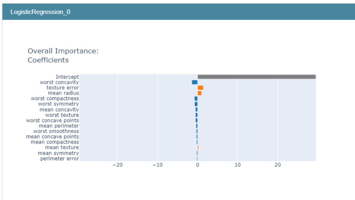
Figura 11. Se muestra la gráfica de explicabilidad global para la regresión logística entrenada con los mismos datos que nosotros. Figura extraída de [23]
