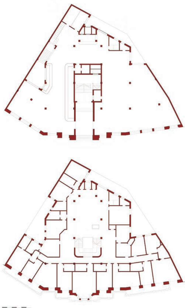
RESTITUCIÓN HIPOTÉTICA DEL HOTEL FLORIDA DE MADRID, OBRA DE ANTONIO PALACIOS RABALO (1922-1924) REALIZADA POR ALVARO BONET EN VERANO DE 2021
