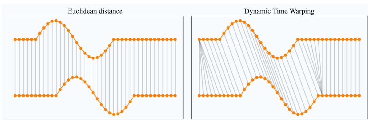
Figura 3.2: Alineamiento de puntos con distancia euclídea y dtw. Imagen de Romain Tavenard [31]
