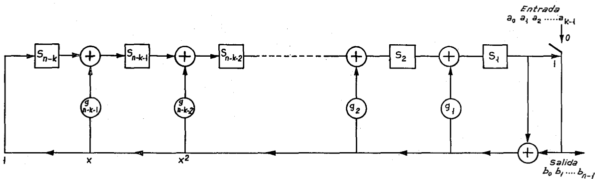
FIG. 2.2. Circuito codificador de (a_0 a_1 \dots a_{k-1}) en (b_0 b_1 \dots b_{n-1}) con estructura separable.
