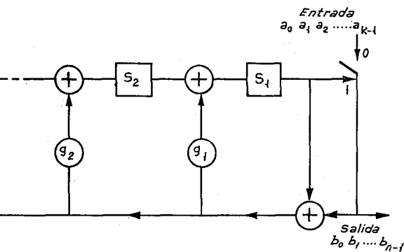
FIG. 2.2. Circuito codificador de (a_0 a_1 \dots a_{k-1}) en (b_0 b_1 \dots b_{n-1}) con estructura separable.
