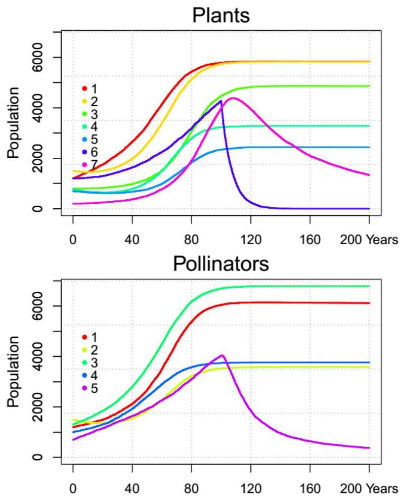
FIGURA 2.16: Quinto experimento. Red débilmente anidada (NODF = 26,39). Una perturbación externa ataca la planta 6. Tabla 2.7.
