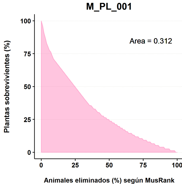
FIGURA 5.2: Curva de destrucción de la red de polinizadores 001 ordenada por MusRank y midiendo la fracción de plantas sobreviviente. El área normalizada bajo la curva es 0.312 (tabla 5.3).
