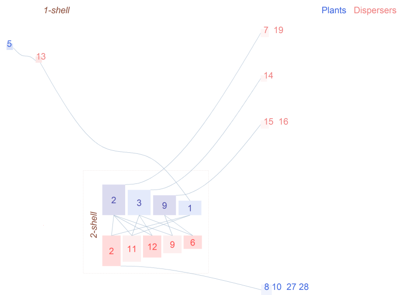
FIGURA 4. 18: Red de frugívoros M_SD_004, en la que se han eliminado todos los polinizadores de la 4-shell, véase la figura 4.6.
