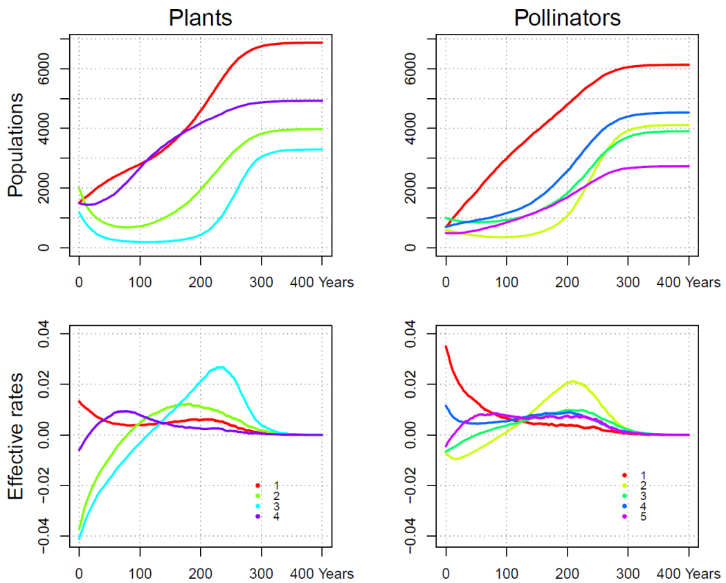
FIGURA 2.12: Resultados del segundo experimento. La configuración puede consultarse en el Anexo 2.8, tabla 2.5.
