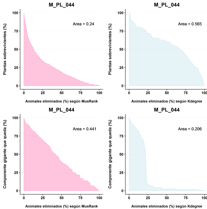
FIGURA 5.5: Rendimiento del procedimiento de extinción de especies animales para MusRank y k_{degree} para las dos magnitudes de salida.
