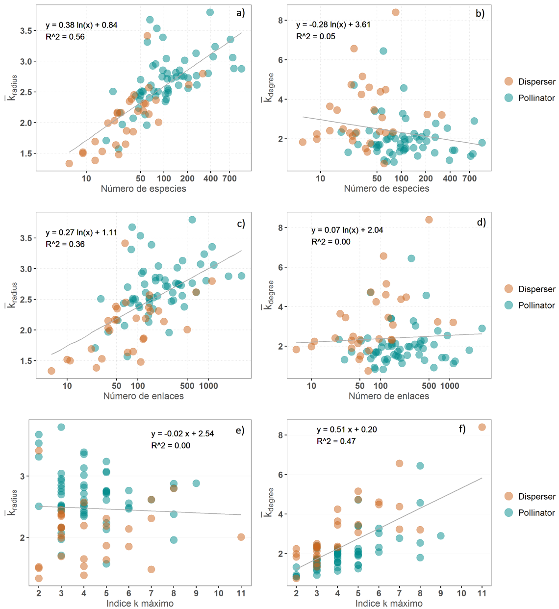
FIGURA 3.7: Diagramas de dispersión que relacionan las k -magnitudes con el tamaño de la red.
