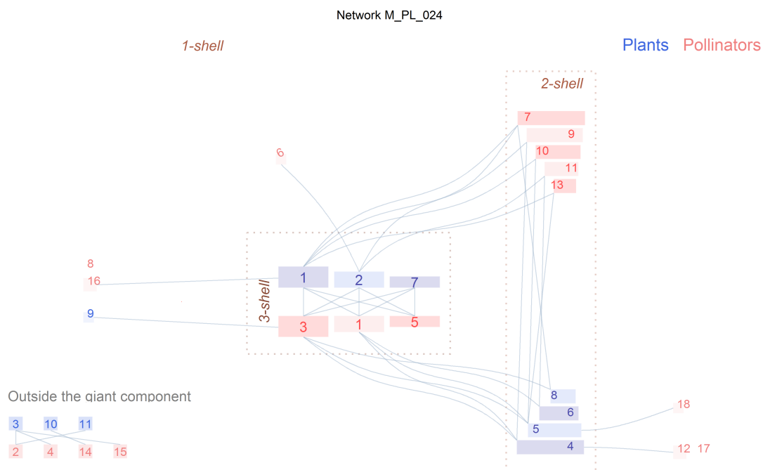
FIGURA 4.7: Red de polinizadores M_PL_024, Melville Island, Canadá [MM67], con 29 especies y 38 enlaces.
