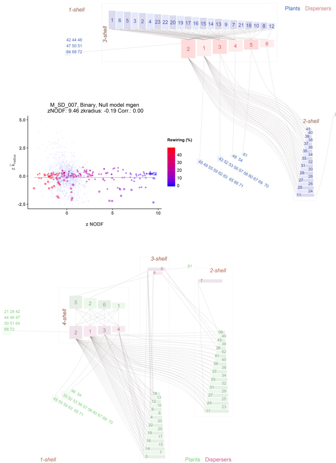
FIGURA 4.16: Red de frugívoros M_SD_007, en el norte de Queensland, Australia [Cro75], con 79 especies y 143 enlaces. Arriba, la red original, \text{NODF} = 51,67 , \bar{k}_{radius} = 2,37 . Abajo, red con seis enlaces recableados al azar, \text{NODF} = 44,75 , \bar{k}_{radius} = 2,09 . En el centro el comportamiento de los índices reducidos ante el proceso de recableado.
