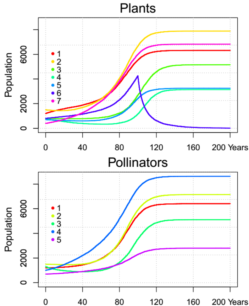
FIGURA 2.14: Cuarto experimento. Red con anidamiento fuerte. Una perturbación externa ataca la especie de planta número 6. Tabla 2.6.
