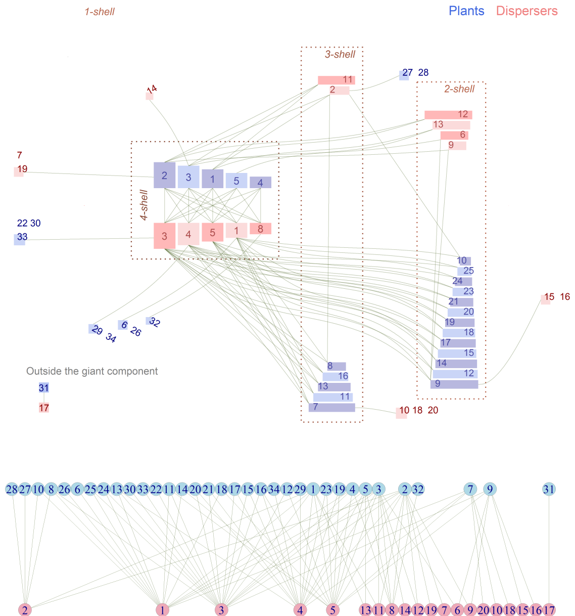
FIGURA 4.6: Diagrama zigurat de una comunidad de aves frugívoras de Puerto Rico M_SD_004, con 54 especies y 95 enlaces [CCG03]. \bar{k}_{radius} = 2,19 ; \bar{k}_{degree} = 2,37 ; NODF = 39,82; Modularity = 0,34. Abajo el diagrama bipartito.
