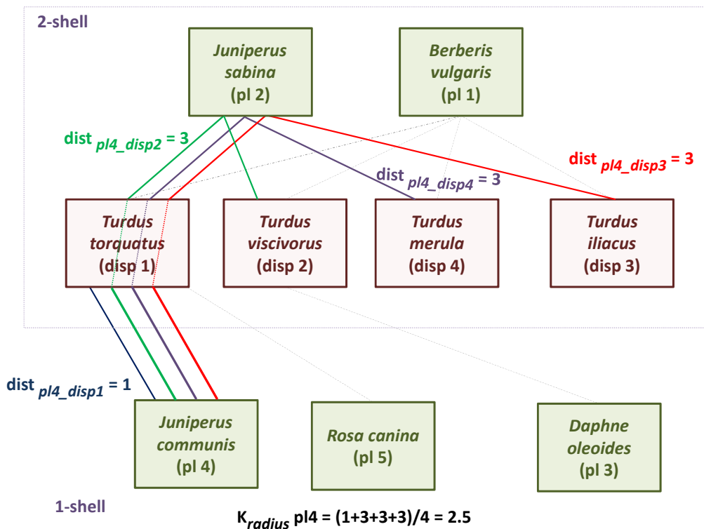
FIGURA 3.3: Cálculo de los k_{radius} de la red de frugívoros en Santa Bárbara, Sierra de Baza (España) [Jor93].
