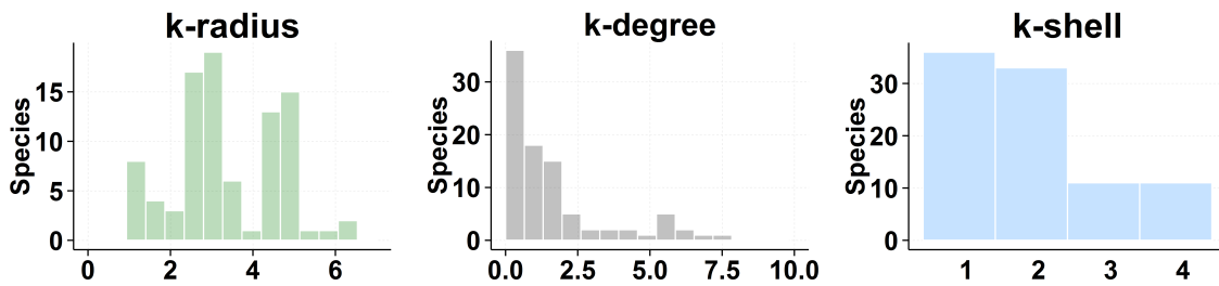
FIGURA 4.9: Histograma de las k magnitudes de polinizadores del Parque Nacional de Canaima, Venezuela [Ram89].
