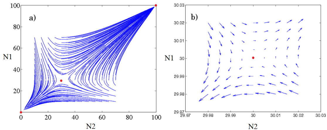
FIGURA 2.3: a) Soluciones del sistema 2.7 para r_1 = r_2 = -0,9 , b_{12} = b_{21} = 0,03 y K_1 = K_2 = 100 . b) Diagrama de flujo en la vecindad del punto de silla en (30,30) .
