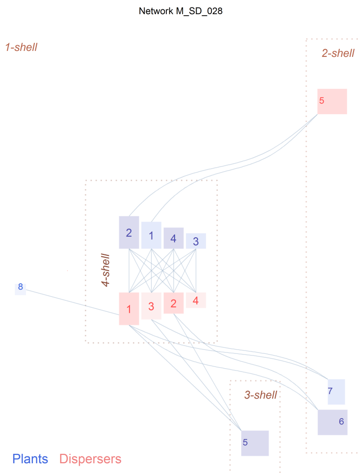
FIGURA 5.1: Diagrama zigurat de una de dispersores en la Cañada Travina, Sierra de Cazorla. Compilada por Pedro Jordano, no publicada.
