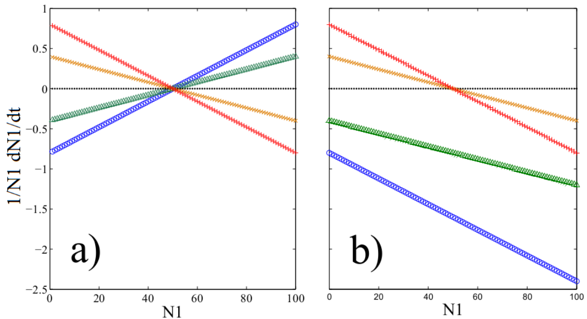
FIGURA 2.1: a) Tasas de crecimiento per cápita para la ecuación logística en la fórmula de Pearl, para las tasas vegetativas r = -0,8 (azul) r = -0,4 (verde), r = 0,4 (naranja) y r = 0,8 (rojo). b) La misma gráfica para la ecuación modificada de nuestro modelo.
