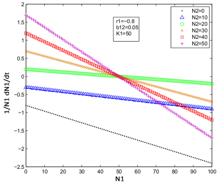
FIGURA 2.2: Crecimiento per cápita de la especie 1 con tasa de crecimiento vegetativa r_1 = -0,8 , capacidad de carga K_1 = 50 , y coeficiente de interacción b_{12} = 0,05 , para diferentes valores de población: N_2 = 0, 10, 20, 30, 40, 50 .
