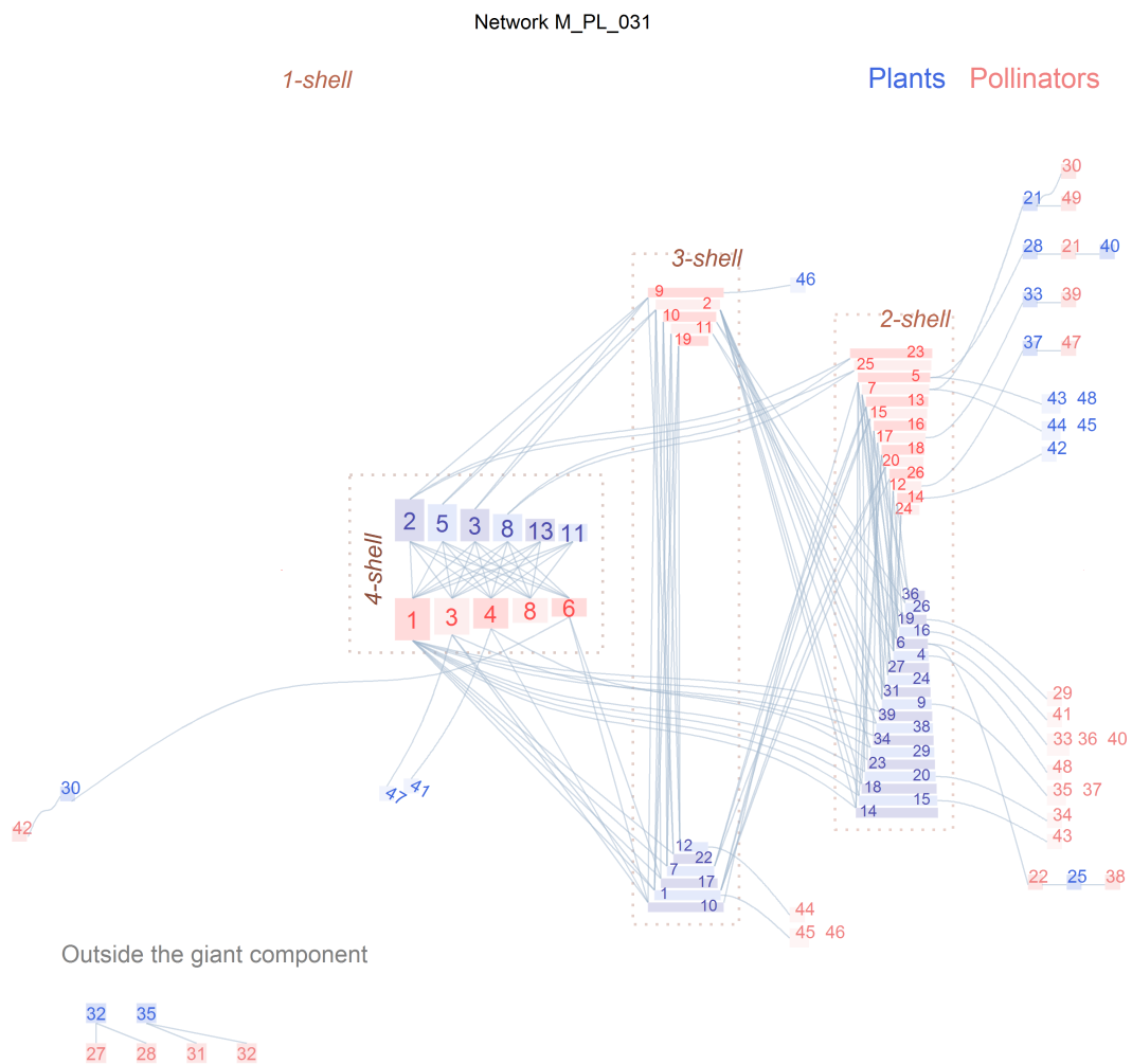
FIGURA 4.8: Red de polinizadores M_PL_031 del Parque Nacional de Canaima, Venezuela, con 97 especies y 156 enlaces [Ram89].
