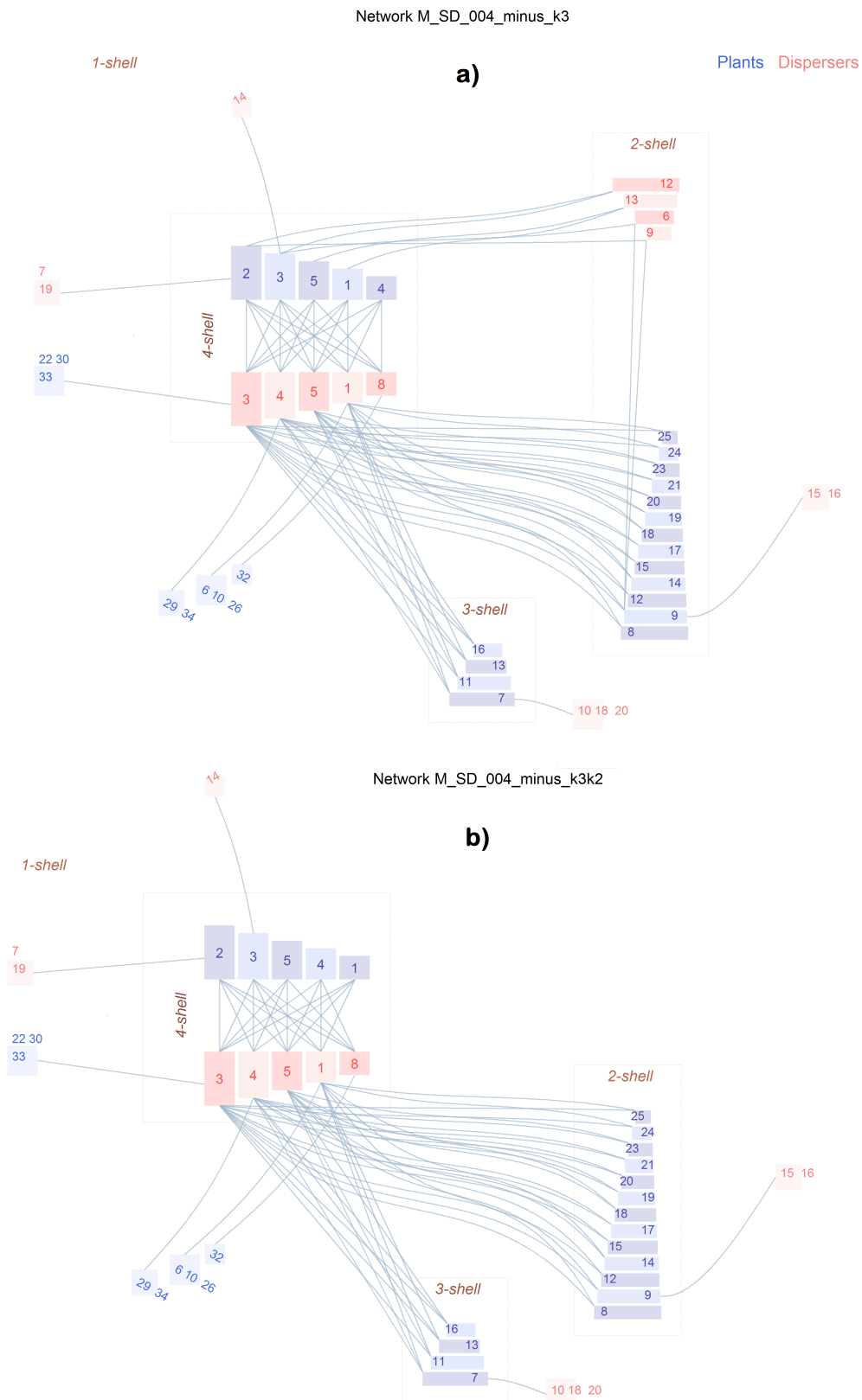
FIGURA 4.21: Red de frugívoros M_SD_004. a: se han eliminado todos los polinizadores de la 3-shell (NODF = 36,24, \bar{k}_{radius} = 2,17 ). b: además se han eliminado los de la 2-shell (NODF = 33,055, \bar{k}_{radius} = 2,15 ), véase la red original en la figura 4.6.
