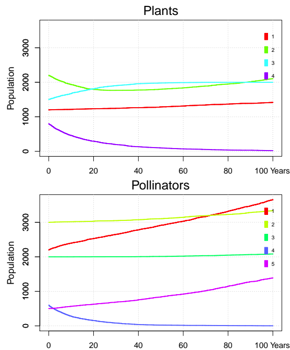
FIGURA 2.10: Resultados del tercer experimento con capacidades de carga constantes. El polinizador 4 y la planta 4 se extinguen. Parámetros en la tabla 2.3.
