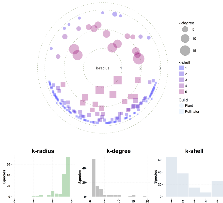
FIGURA 4.3: Diagrama polar de una comunidad de polinizadores en la isla de Chiloé (Chile) [SR+05].
