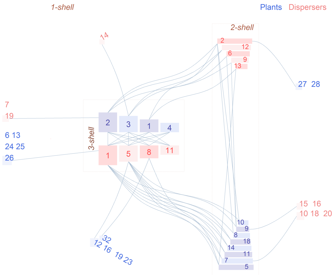
FIGURA 4.17: Red de frugívoros M_SD_004, en la que se han eliminado los polinizadores números 3 y 4, los dos de mayor k_{degree} , véase la figura 4.6.
