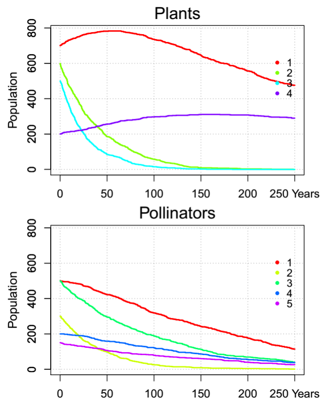
FIGURA 2.11: Resultados del primer experimento. La parametrización puede verse en el Anexo 2.8, tabla 2.4.
