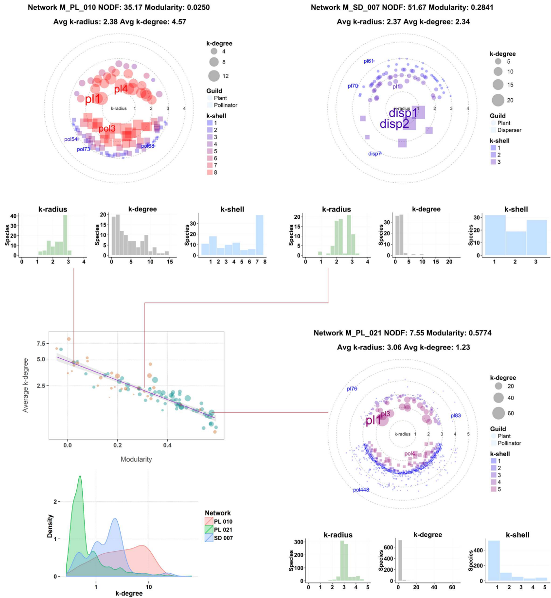
FIGURA 4.4: Comparación de tres redes mediante sus diagramas polares.
