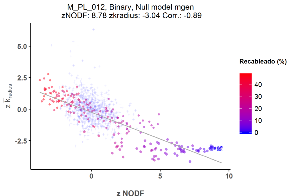
FIGURA 3.5: Gráfica del experimento de recableado para la red de polinizadores número 12 (Parque de Garajonay, compilada por Olesen, no publicada). La nube de cruces pequeñas representa los pares de valores zNODF, z\bar{k}_{radius} de las 1000 realizaciones del modelo nulo. Los puntos representan ese par de valores para cada red recableada. El aspa azul dentro de un círculo señala los valores de zNODF, z\bar{k}_{radius} de la red original. La recta gris, el resultado de la regresión lineal para los valores de las redes recableadas.
