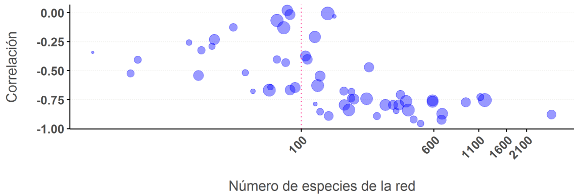
FIGURA 3.13: Correlación de z\bar{k}_{radius} y zNODF en el experimento de recableado en función del número de especies de la red. El área es proporcional a la asimetría de clases de cada red.
