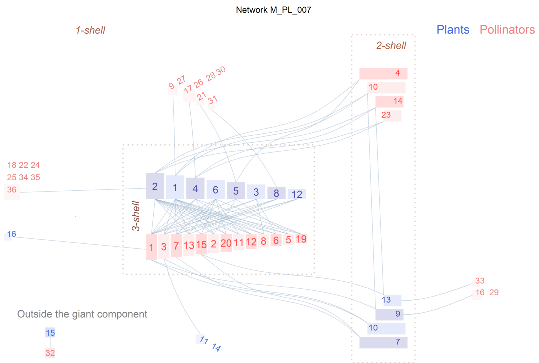
FIGURA 5.6: Red de polinizadores en Shelfanger, Norfolk, Reino Unido [DCP02].
