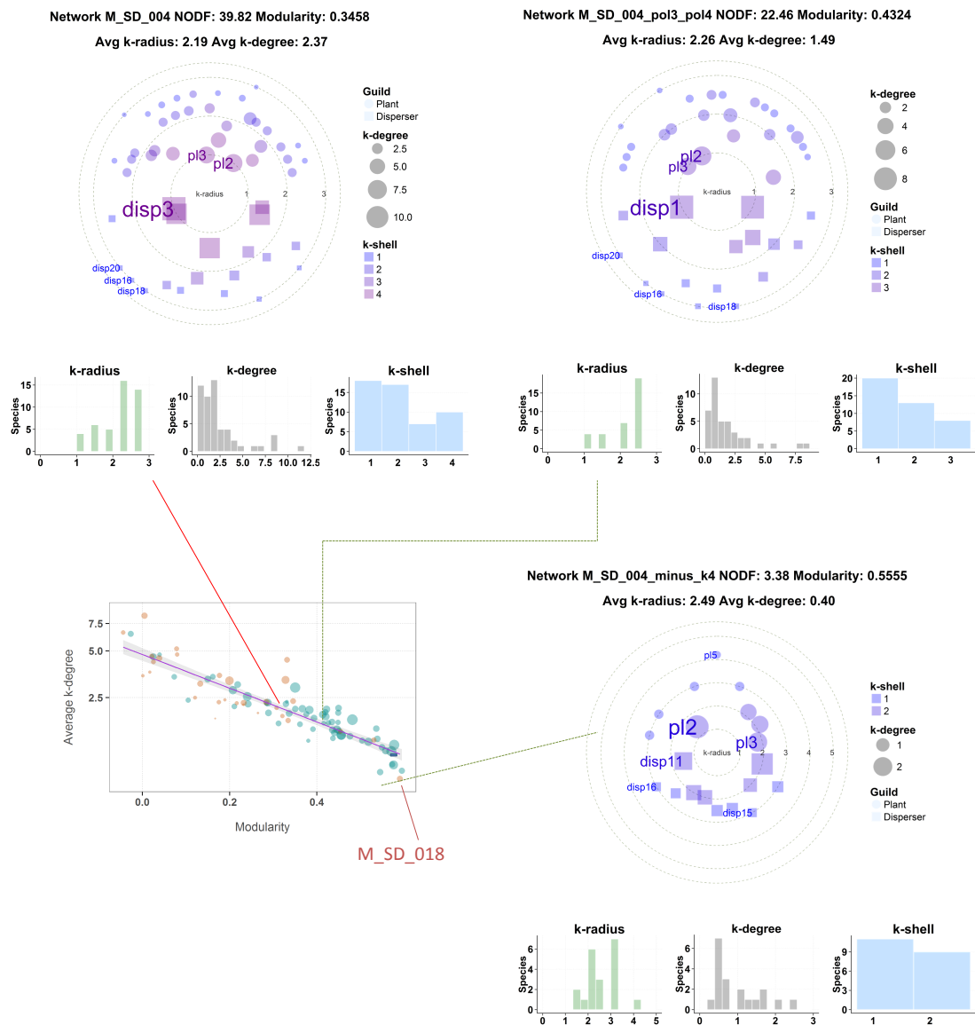
FIGURA 4.20: Diagramas polares de la red M_SD_004 intacta, tras eliminar los dos polinizadores de mayor k_{degree} y tras suprimir la 4-shell de polinizadores completa.
