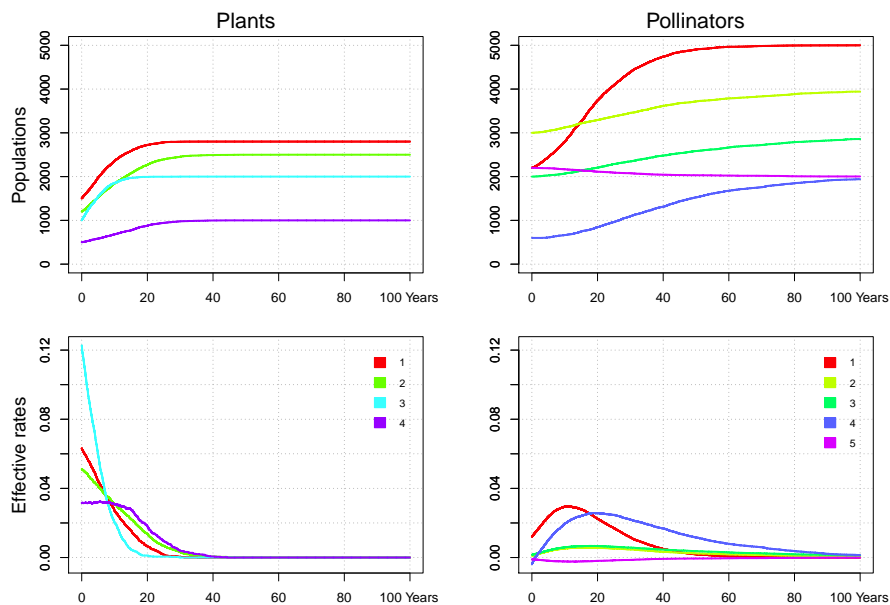
FIGURA 2.9: Segundo experimento. Evolución temporal de las poblaciones y de las tasas de crecimiento efectivas del mismo sistema de 4 + 5 especies (figura 2.7). La comunidad termina con todas las especies en sus capacidades de carga respectivas. Parámetros en la tabla 2.2.
