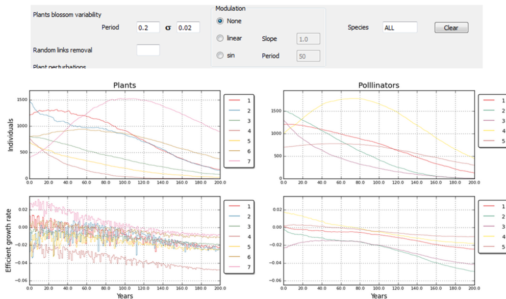
FIGURA A.8: Perturbación gaussiana en el periodo de floración con desviación estándar constante.
