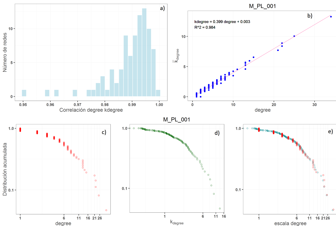
FIGURA 3.8: Relación entre degree y k_{\text{degree}} . a: histograma de la correlación entre ambas magnitudes para todas las redes del estudio (a); b: diagrama de dispersión de ambas magnitudes para la red de polinizadores 001 y valores de la regresión lineal para esta red; c,d,e: distribuciones de probabilidad acumulada de los dos índices. En e) se han representado ambos sobre la escala de degree, con la transformación en el eje X k_{\text{degree}} = \alpha * \text{degree} , siendo \alpha el coeficiente de regresión lineal que en este caso vale aproximadamente 0,4.
