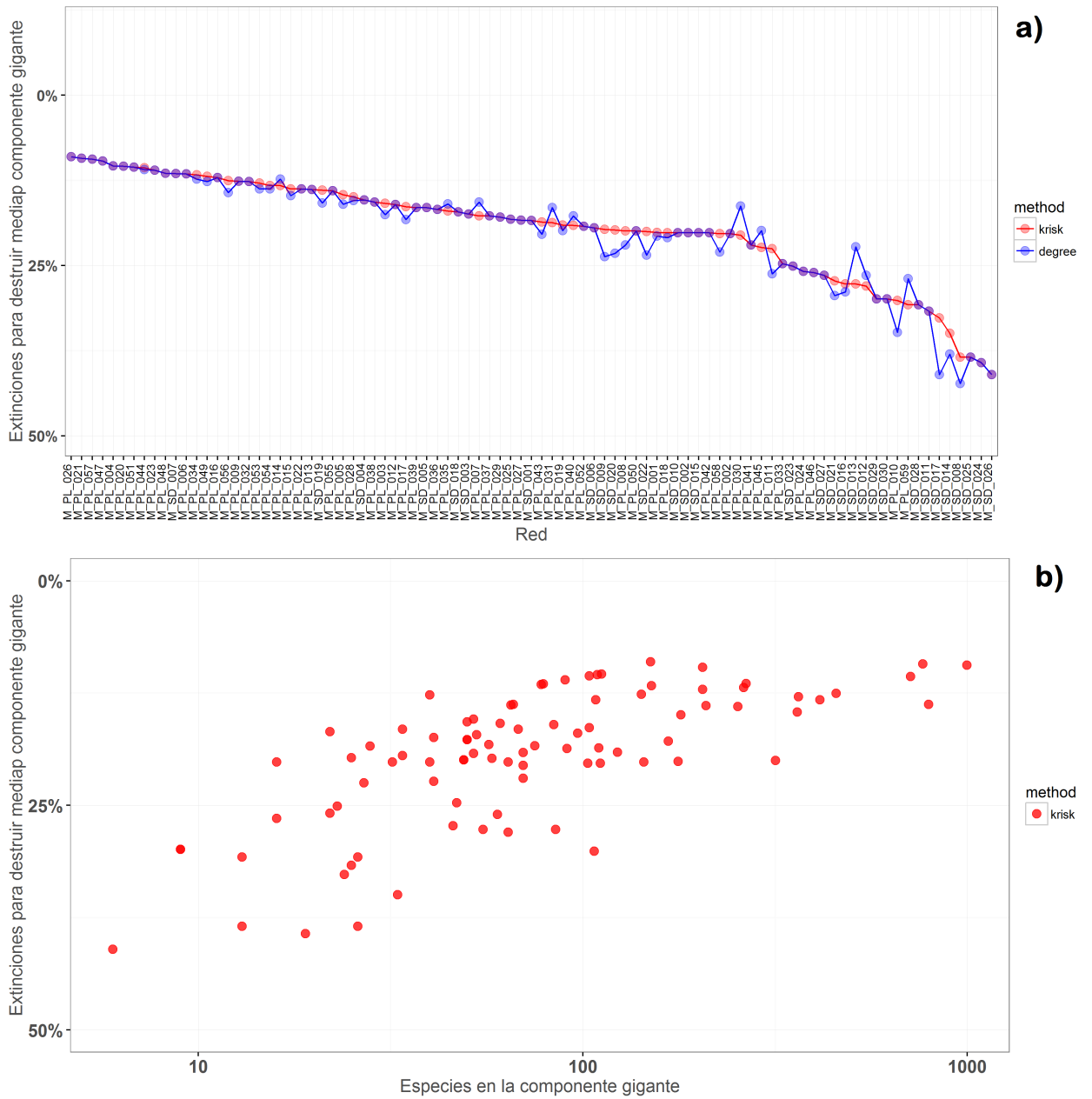
FIGURA 5.4: Comparación del rendimiento de los dos criterios más destructivos de la mitad de la componente gigante, k_{risk} y degree (a) y comportamiento de k_{risk} en función del tamaño de la red (b).
