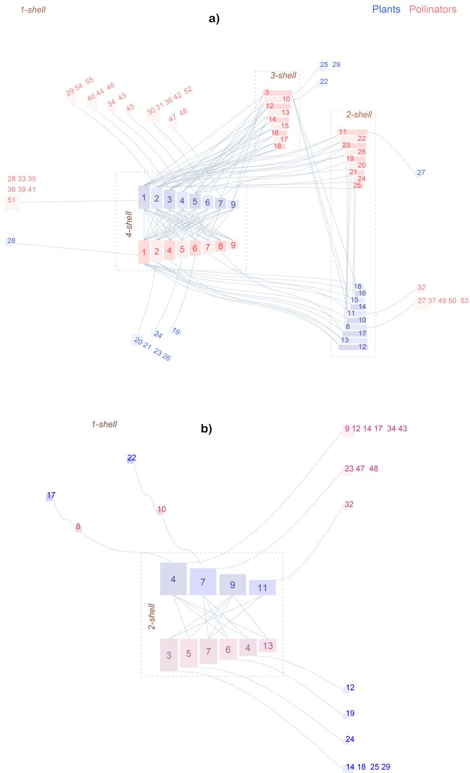
FIGURA 5.3: Destrucción de la componente gigante de la red de polinizadores número 012 (Olesen, no publicada), ordenando por k_{risk} . Red original con 84 especies (a). Componente gigante que queda tras retirar las 7 especies más importantes, siguiendo esta secuencia: planta1, planta2, polinizador2, polinizador1, planta3, planta6 y planta5 (b).
