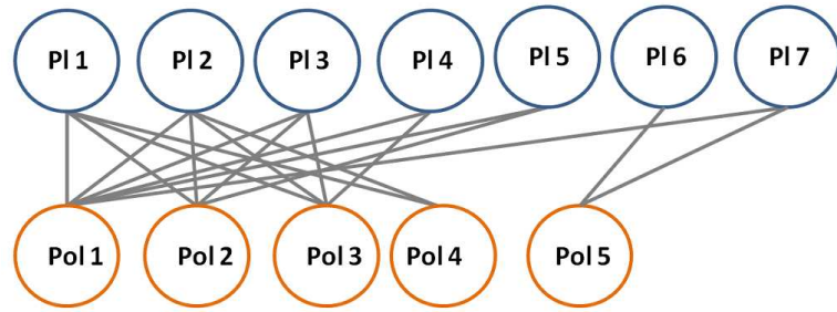
FIGURA 2.15: Red débilmente anidada (NODF = 26,39). Tabla 2.7.
