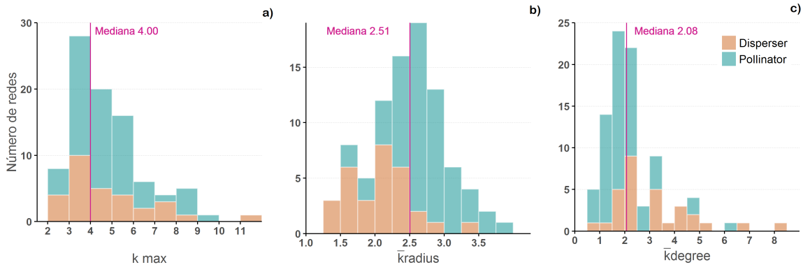
FIGURA 3.6: Histogramas de las k -magnitudes de las 89 redes de la colección.
