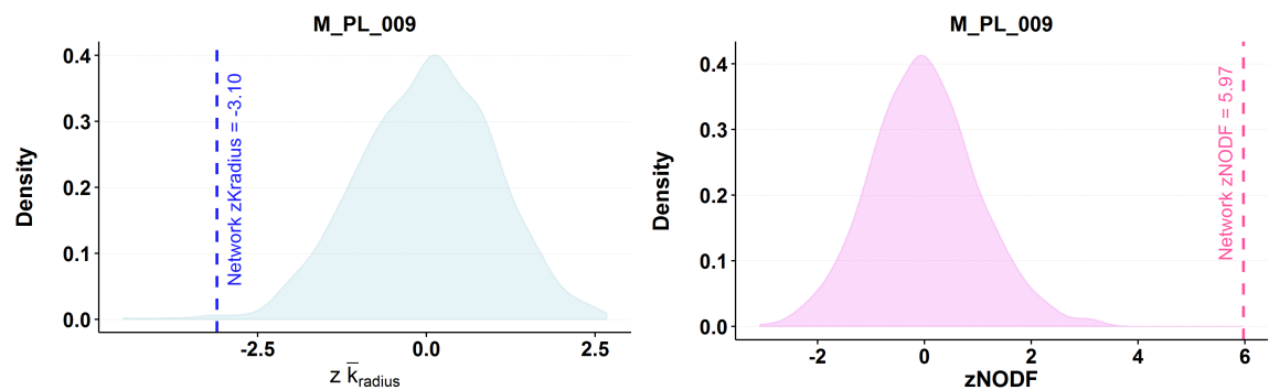
FIGURA 3.4: Ejemplo de z scores de \bar{k}_{\text{radius}} y NODF para una red de polinizadores con matriz de adyacencia binaria [EO99].
