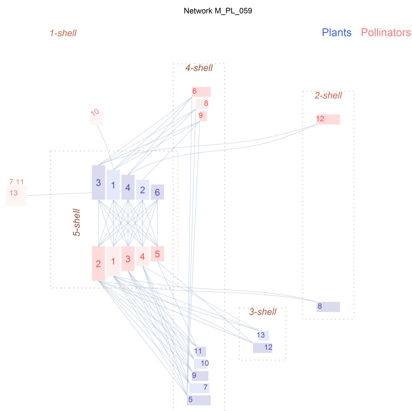
FIGURA 4.13: Red de polinizadores M_PL_059, Parque Nacional do Catimbau, Brasil, con 26 especies y 71 enlaces [BMM09]. NODF = 76,88 , \bar{k}_{radius} = 1,57 .
