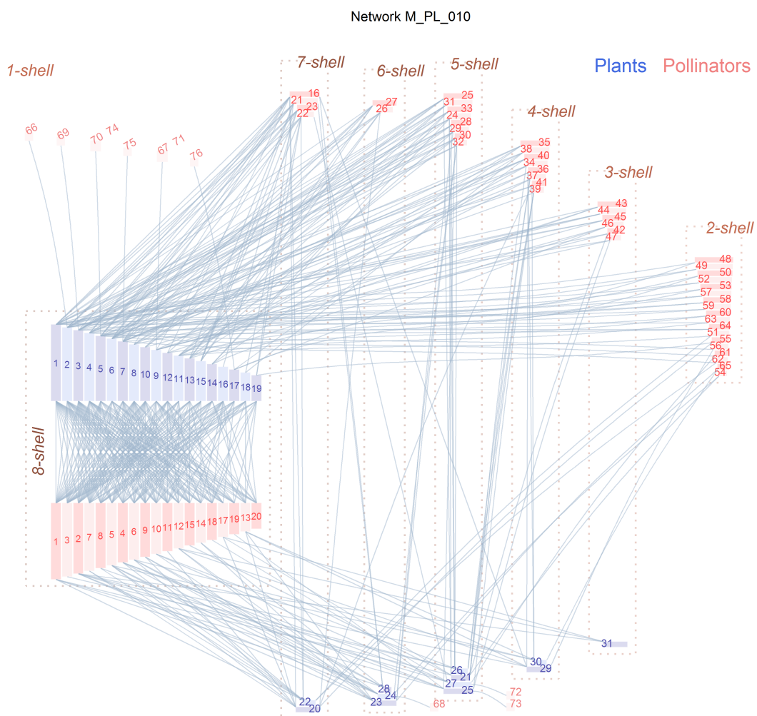
FIGURA 4.10: Red de polinizadores M_PL_010 (Elberling & Olesen, no publicada), con 107 especies y 456 enlaces. Su diagrama polar puede verse en la figura 4.4.
