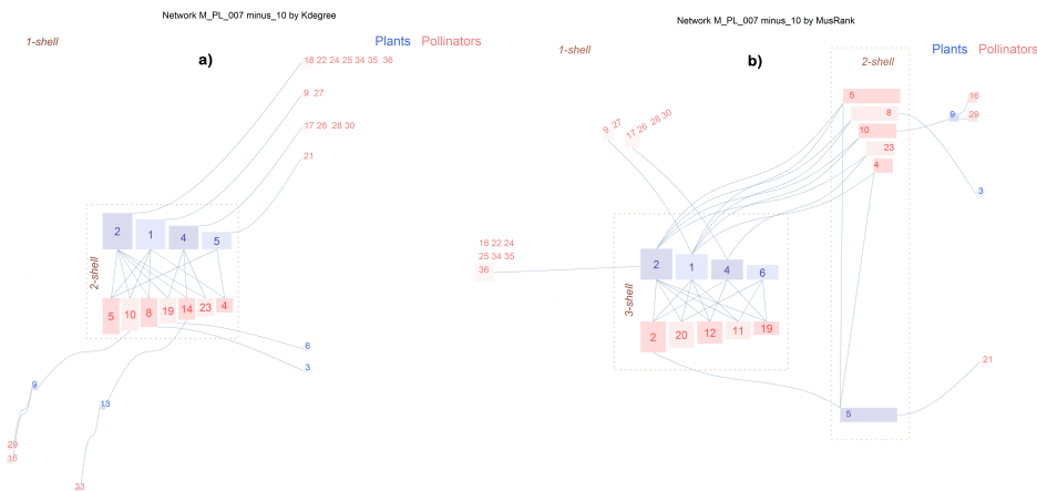
FIGURA 5.7: Resultado de la retirada de 10 especies animales de la red M_PL_007 . Siguiendo el orden indicado por k_{degree} (a). La componente gigante que queda tiene 32 especies (8 de plantas, 24 de polinizadores). Siguiendo MusRank (b). La componente gigante tiene 33 especies (7 de plantas, 26 de polinizadores).
