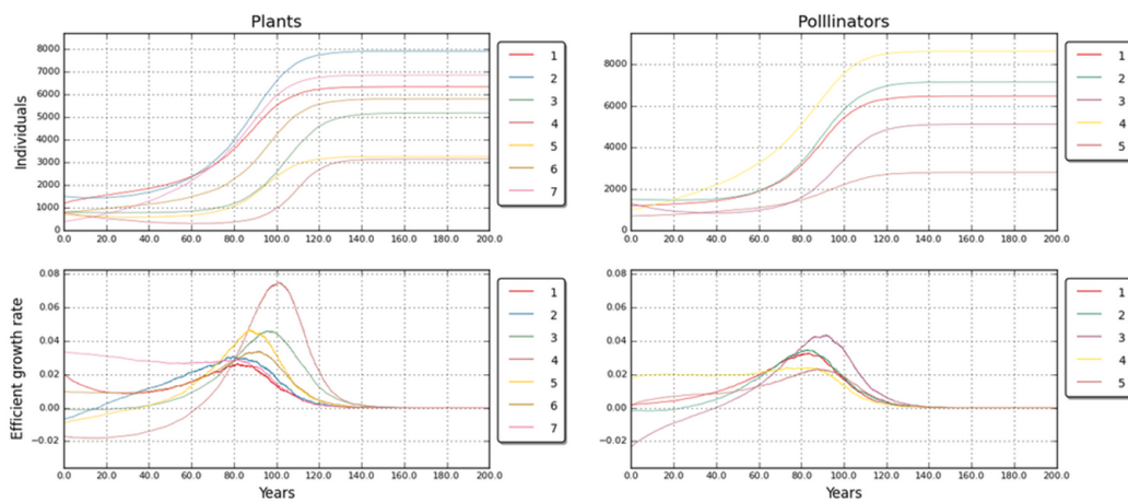
FIGURA A.6: Evolución dinámica sin perturbaciones en la red ejemplo.
