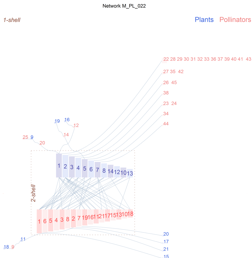
FIGURA 4.14: Red de polinizadores M_PL_022, Los Andes, Argentina, con 66 especies y 83 enlaces [Med+02]. NODF = 18,02 , \bar{k}_{radius} = 3,68 .
