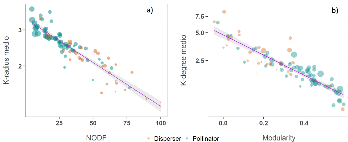
FIGURA 3.9: Diagrama de dispersión del \bar{k}_{\text{radius}} respecto a NODF (a), y del \bar{k}_{\text{degree}} respecto a la Modularity (b). Cada punto es una red, su área es proporcional al logaritmo del número de especies y el color indica la clase de comunidad. Se han incluido las líneas de regresión con sus intervalos de confianza en sombreado.
