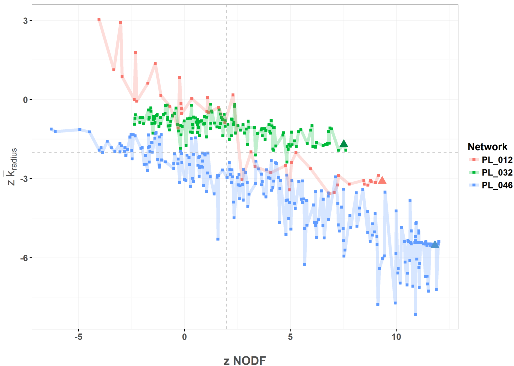
FIGURA 3.14: Comparativa de la evolución de z\bar{k}_{\text{radius}} y z\text{NODF} en el experimento de recableado de tres redes. Los triángulos marcan los pares de valores de las redes originales. A medida que crece el porcentaje de recableado aleatorio, las redes resultantes son más desordenadas y se desplazan al cuadrante superior izquierdo, combinación de falta de anidamiento y de compacidad.
