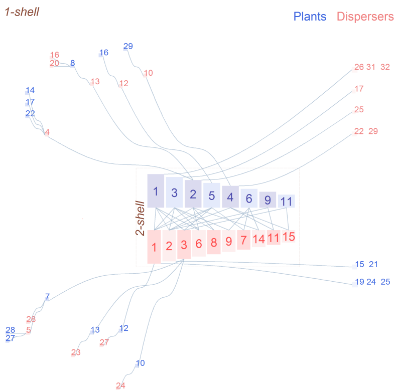
FIGURA 4. 19: Red de frugívoros M_SD_018, en Papúa Nueva Guinea [MW96].
