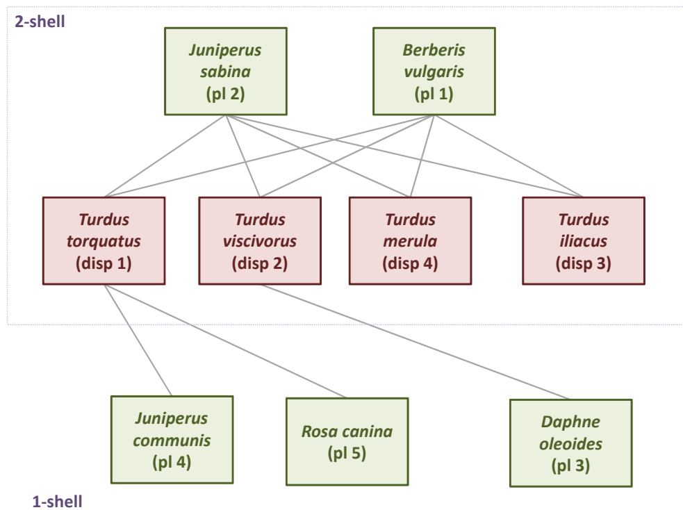
FIGURA 3.2: Red de frugívoros en Santa Bárbara, Sierra de Baza (España) [Jor93].
