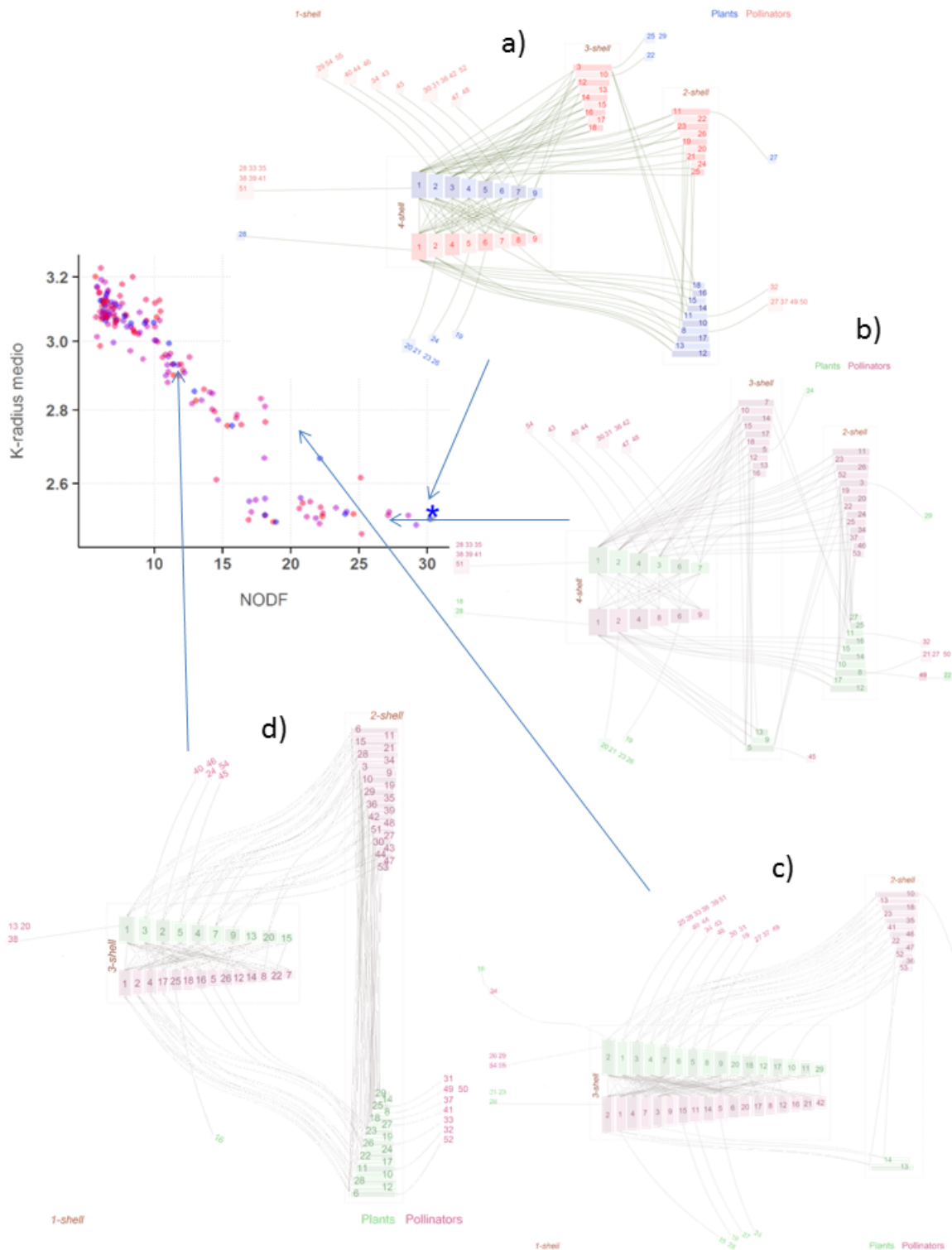
FIGURA 4.15: Red de polinizadores M_PL_012, en el Parque Nacional de Garajonay, La Gomera (España), compilada por Olesen y no publicada, con 84 especies y 145 enlaces. a: red original, NODF = 30,40, \bar{k}_{radius} = 2,51 . b: red con siete enlaces recableados al azar, NODF = 26,62, \bar{k}_{radius} = 2,48 . c: con diecisiete enlaces recableados, NODF = 22,62, \bar{k}_{radius} = 2,77 . d: con treinta y dos, NODF = 13,22, \bar{k}_{radius} = 2,82 .
