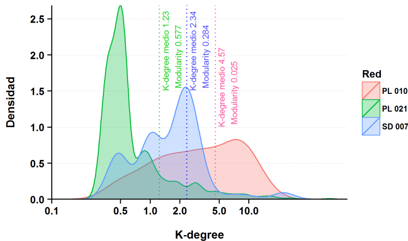
FIGURA 3.10: Distribución de densidad del k_{degree} en tres redes diferentes. Junto a las líneas verticales pueden verse los valores del \bar{k}_{degree} y de la Modularity.
